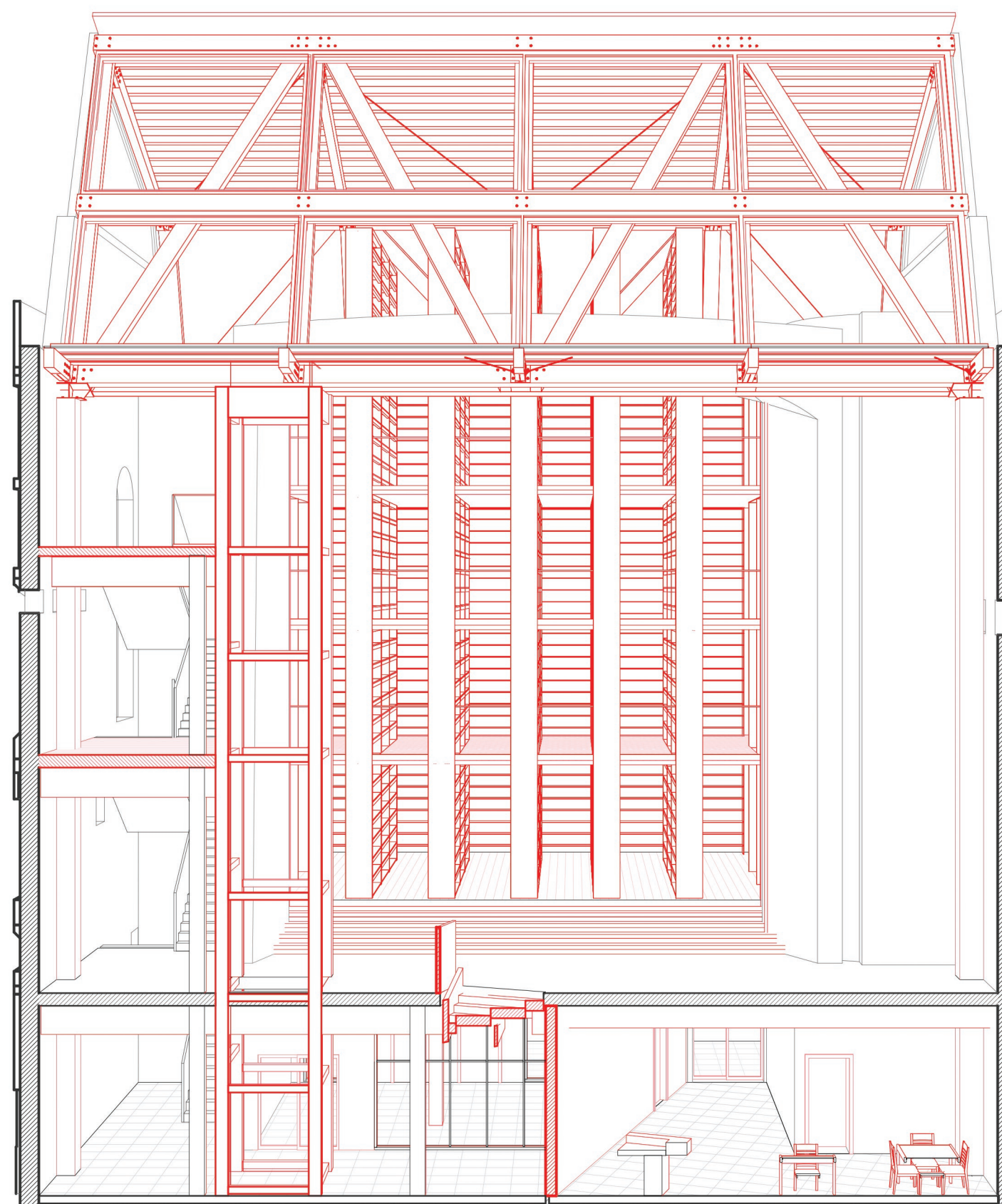
CORTE TRANSVERSAL NORTE
