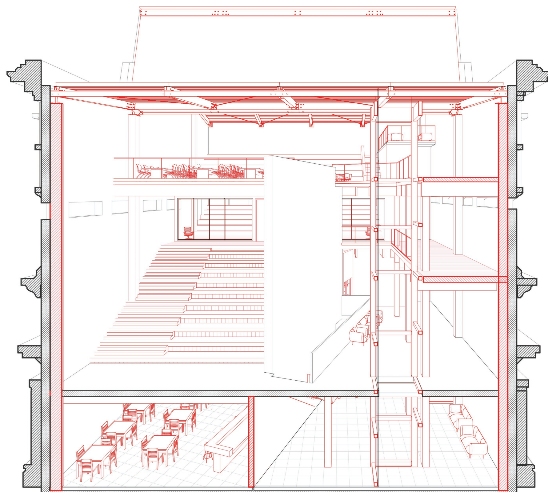
CORTE TRANSVERSAL SUR
