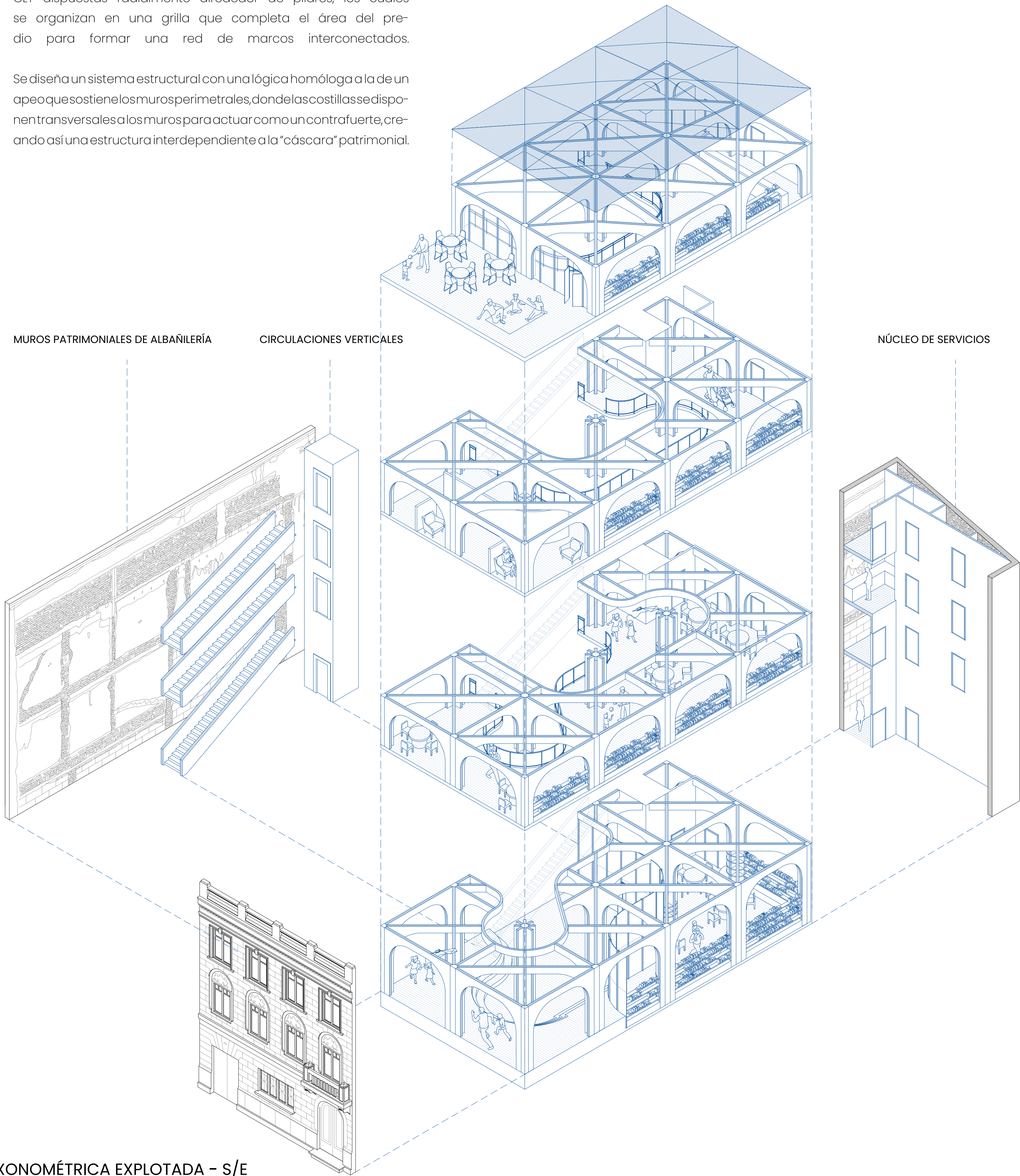
AXONOMÉTRICA EXPLOTADA - S/E
