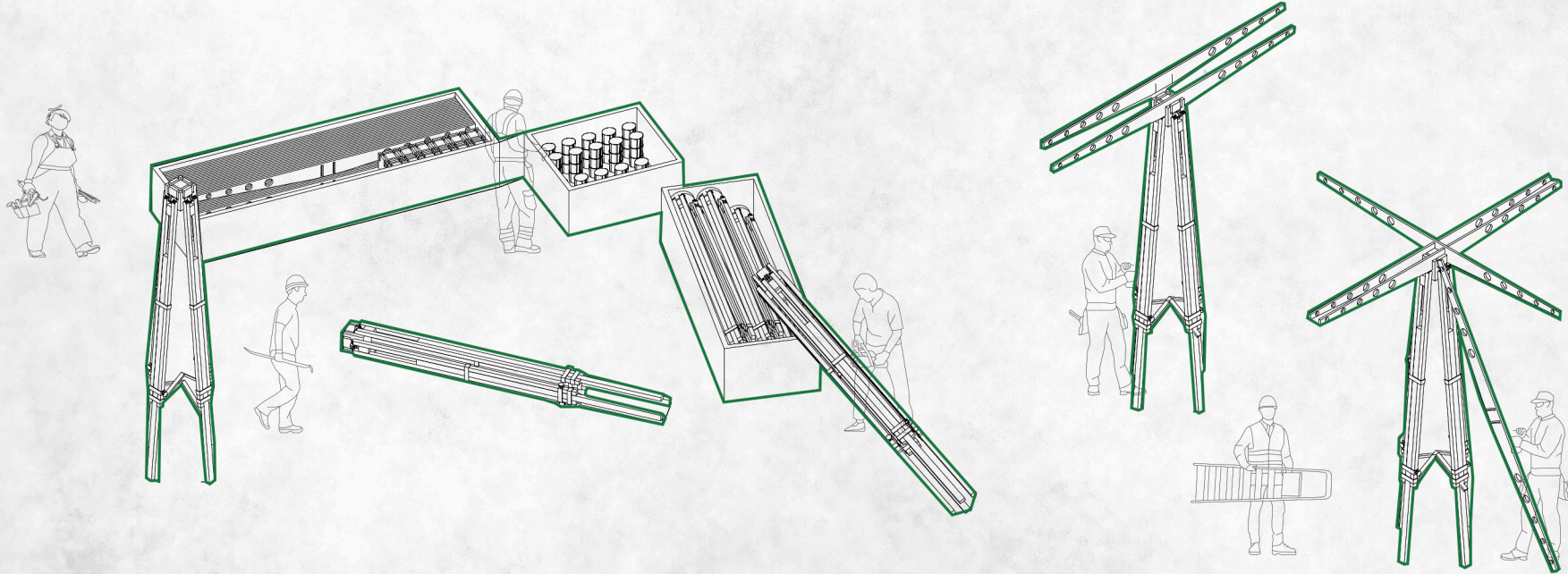
APERTURA DE CAJAS Y POSICIONAMIENTO DE TETRÁPODOS
