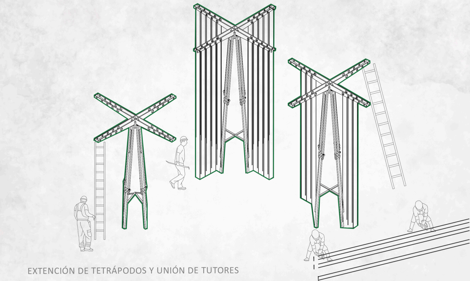
EXTENSIÓN DE TETRÁPODOS Y UNIÓN DE TUTORES
