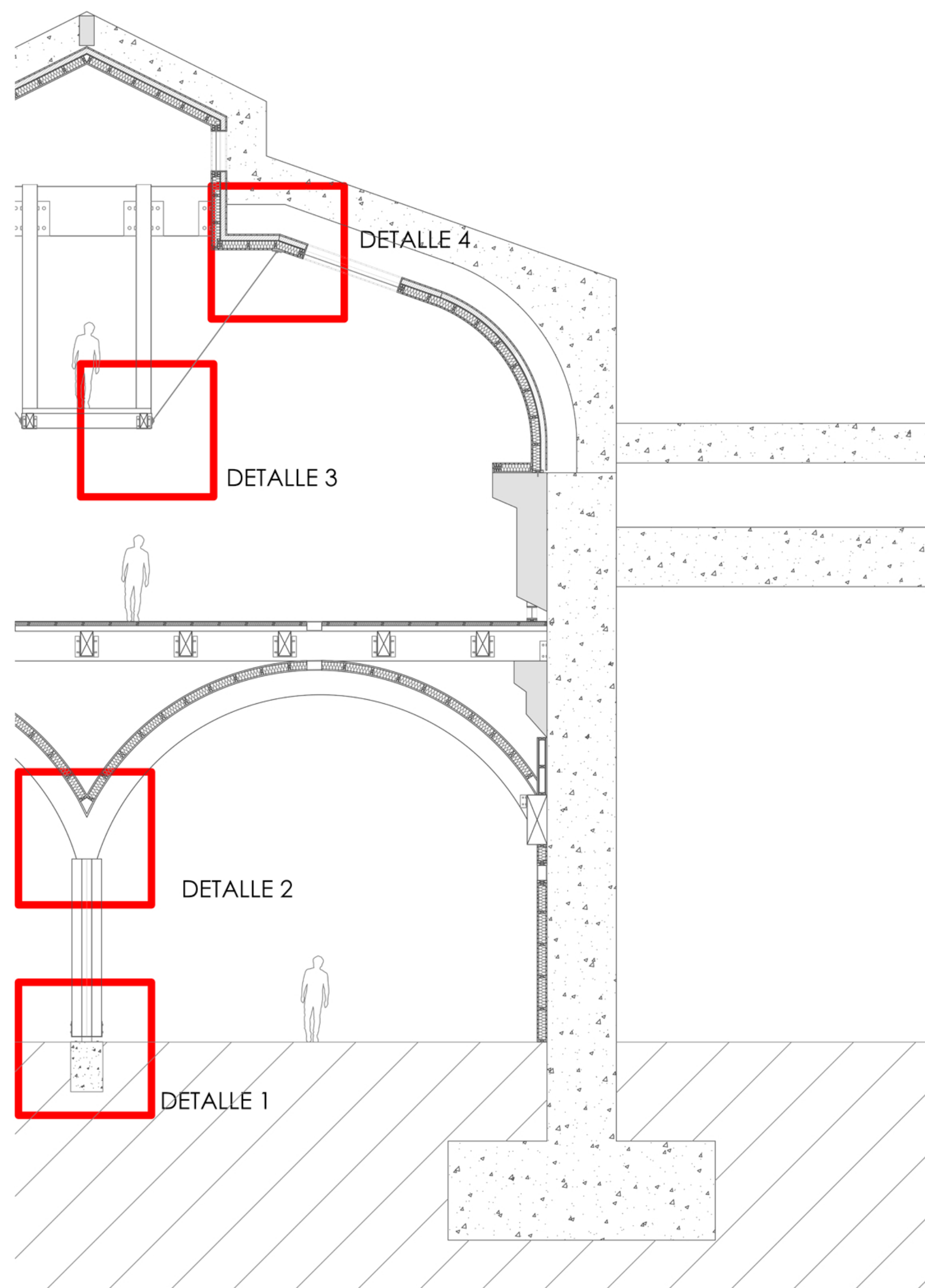
ESCANTILLÓN ESC 1:75
