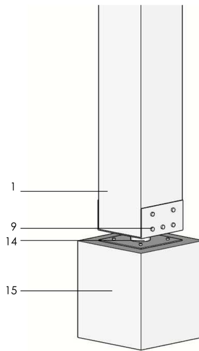
DETALLE 1 PIE DE PILAR ESC 1:10
