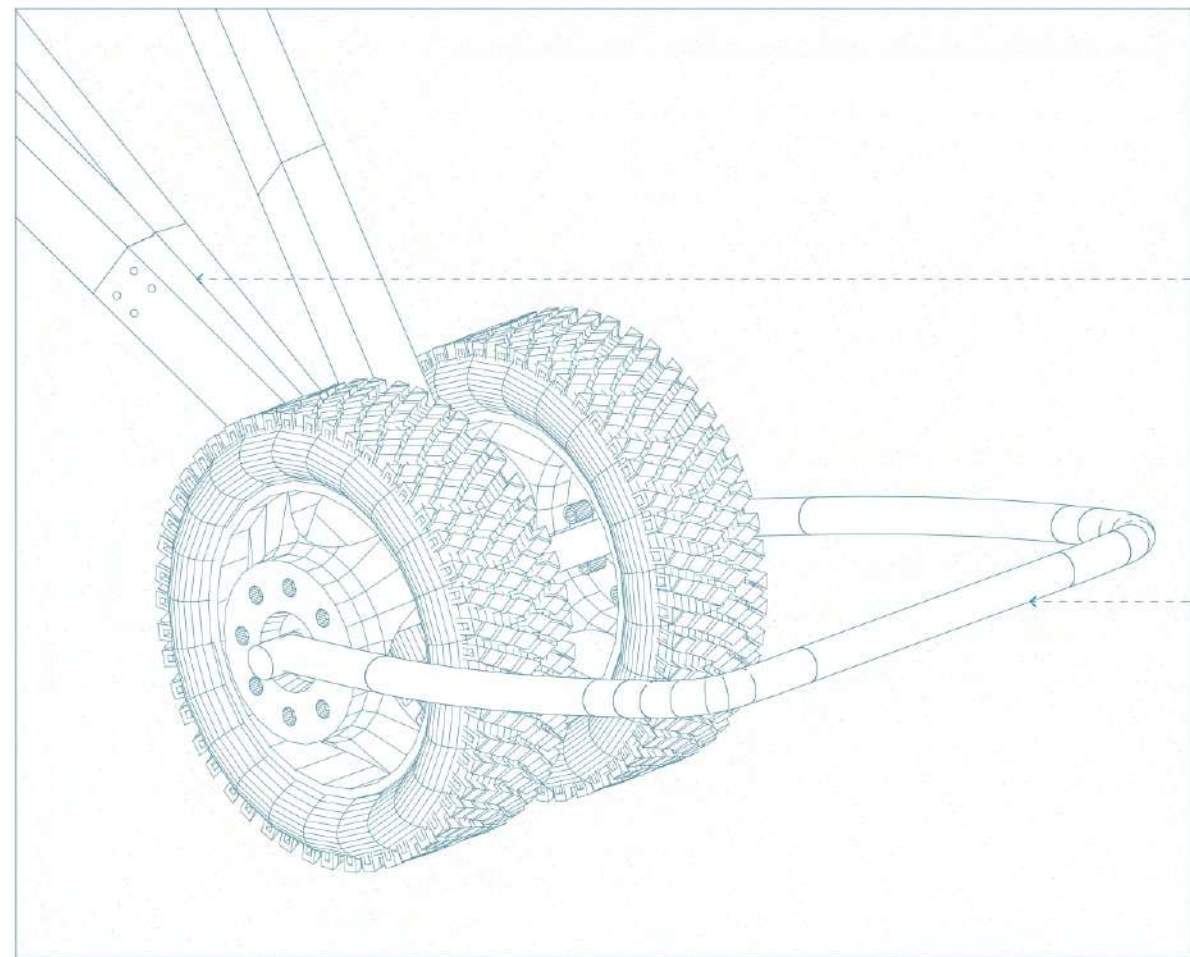
D4 UNION DE RUEDAS A MODULO
