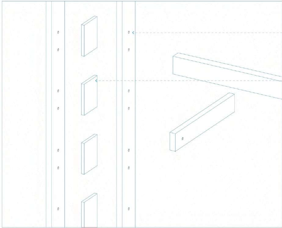
D2 PILAR SOPORTE COMPUESTO
