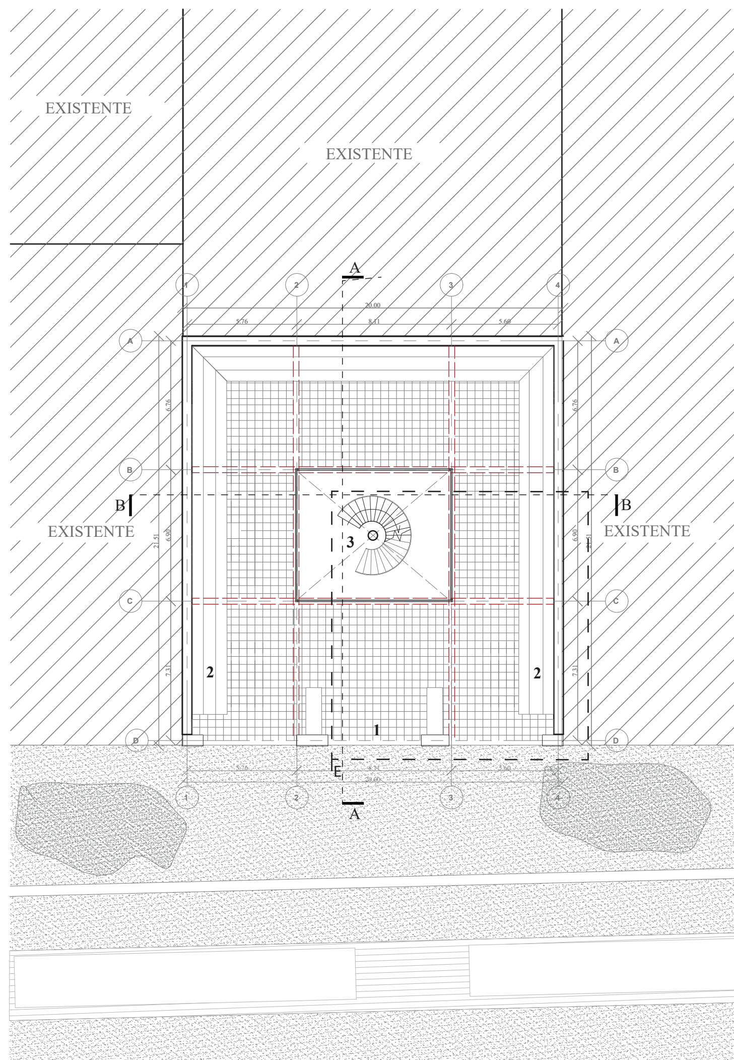
PLANTA NIVEL 1 Escala: 1:200
