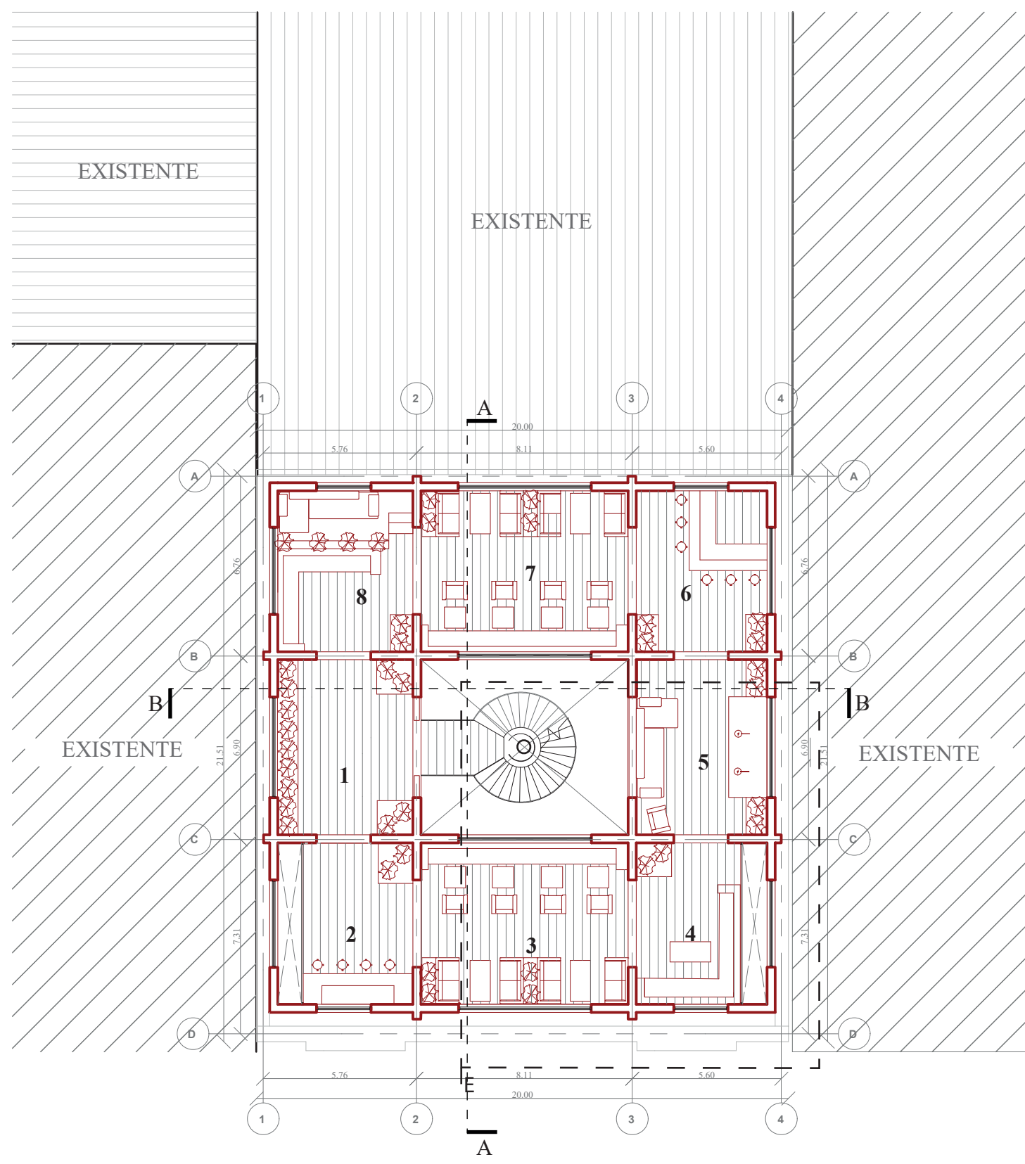
PLANTA NIVEL 4 Escala: 1:200
