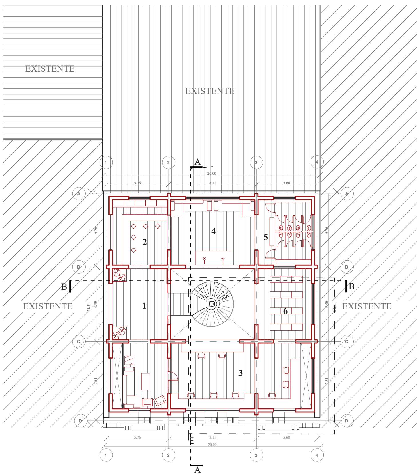
PLANTA NIVEL 3 Escala: 1:200
