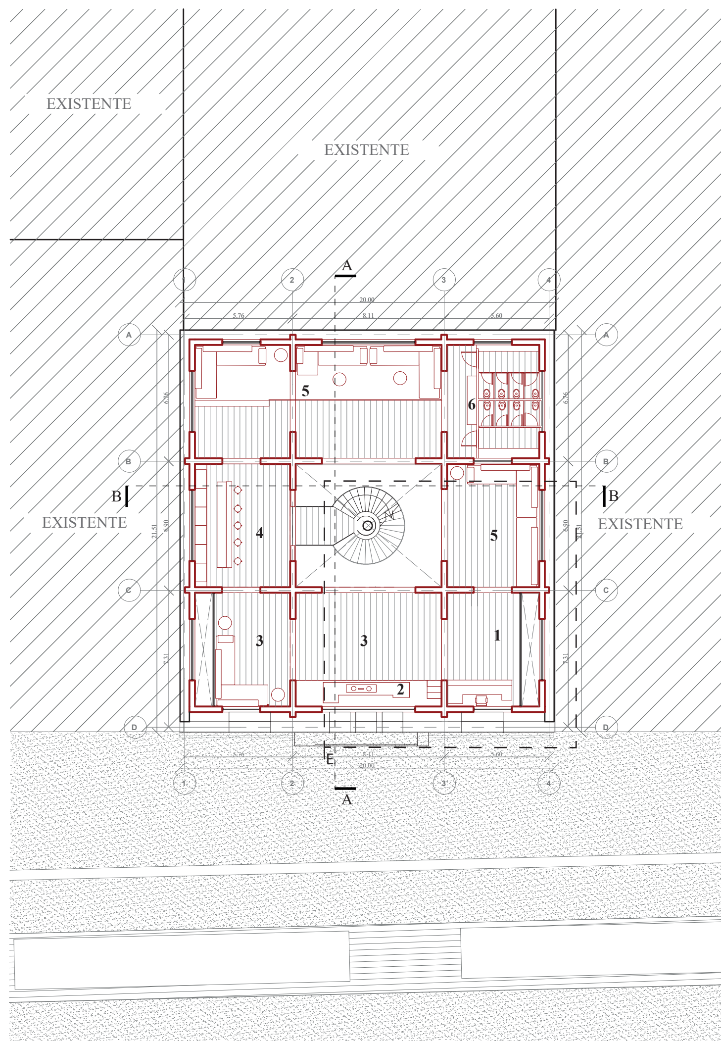
PLANTA NIVEL 2 Escala: 1:200
