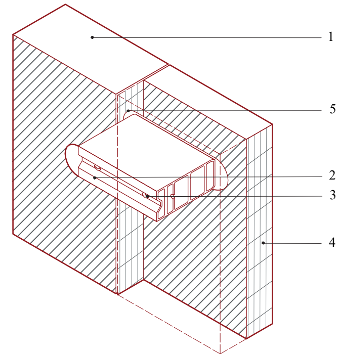
DETALLE 3 UNIÓN PANELES CLT ESC. 1:20
