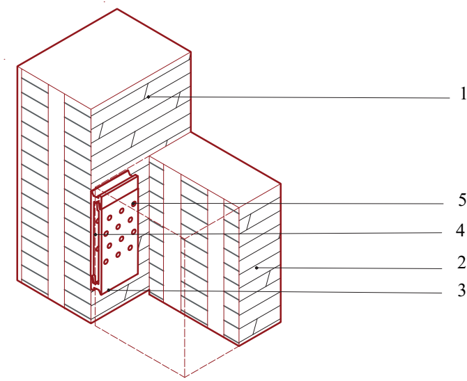
DETALLE 1 UNIÓN PISO-MURO CLT ESC. 1:20
