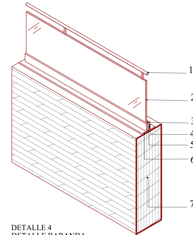
DETALLE 4 DETALLE BARANDA ESC. 1:20
