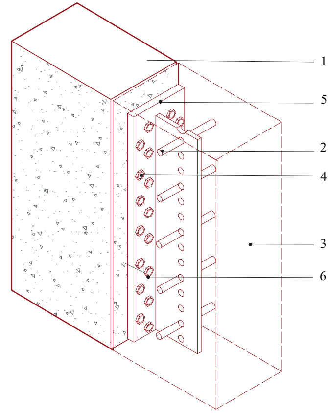
DETALLE 2 UNIÓN MEDIANERO-CLT ESC. 1:20
