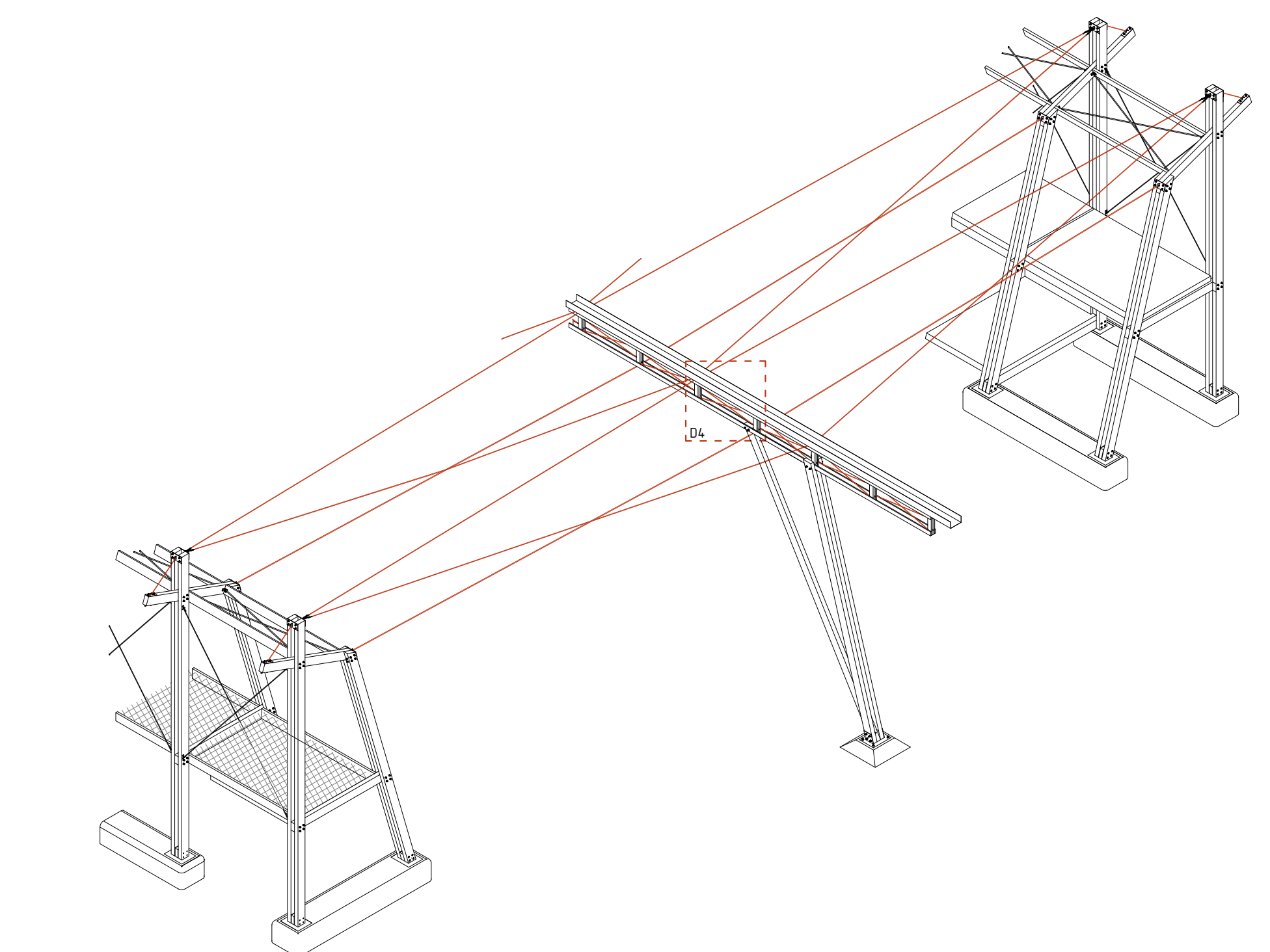
AXONOMETRICA UNIÓN MODULO - CUBIERTA
