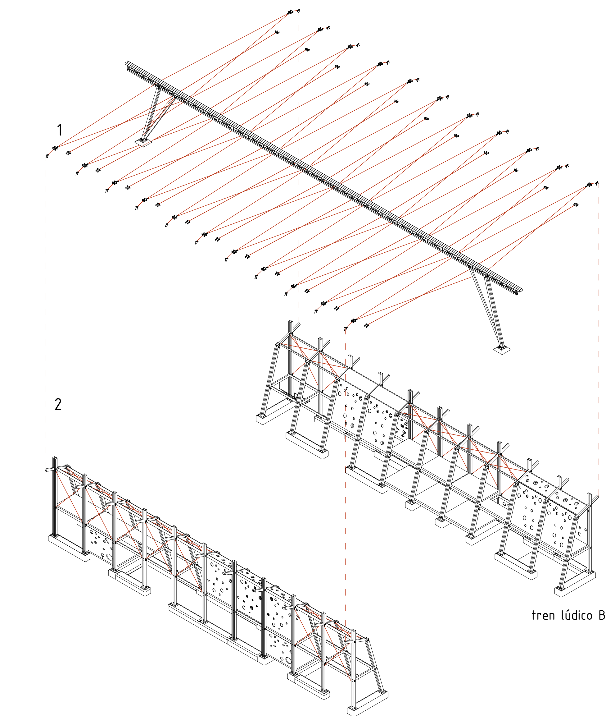
01 Cubierta 02 Estructura
