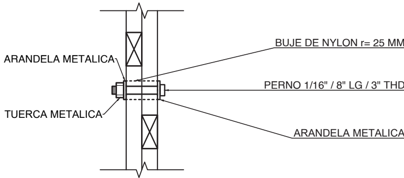
SECCION 1-1 - ARRIOSTRAMIENTO MÓVIL Esc. 1/10 - COTAS EN CM
