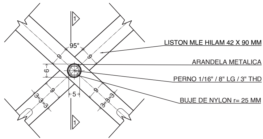
DETALLE 1 - ARRIOSTRAMIENTO MÓVIL Esc. 1/10 - COTAS EN CM
