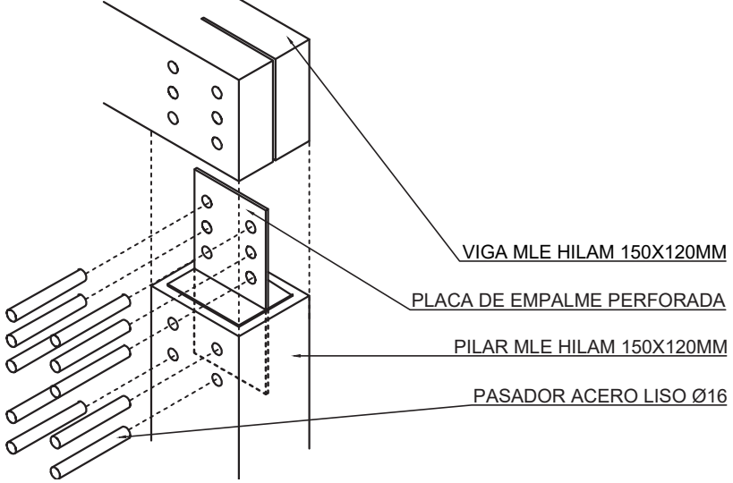
DETALLE 3 - UNIONES MARCO MLE Esc. 1/10
