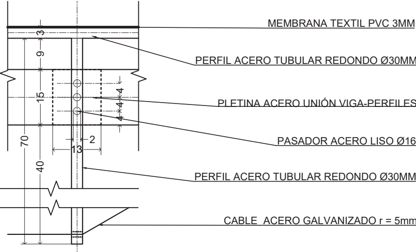
DETALLE 2 - ENVOLVENTE Y TENSORES Esc. 1/10 - COTAS EN CM
