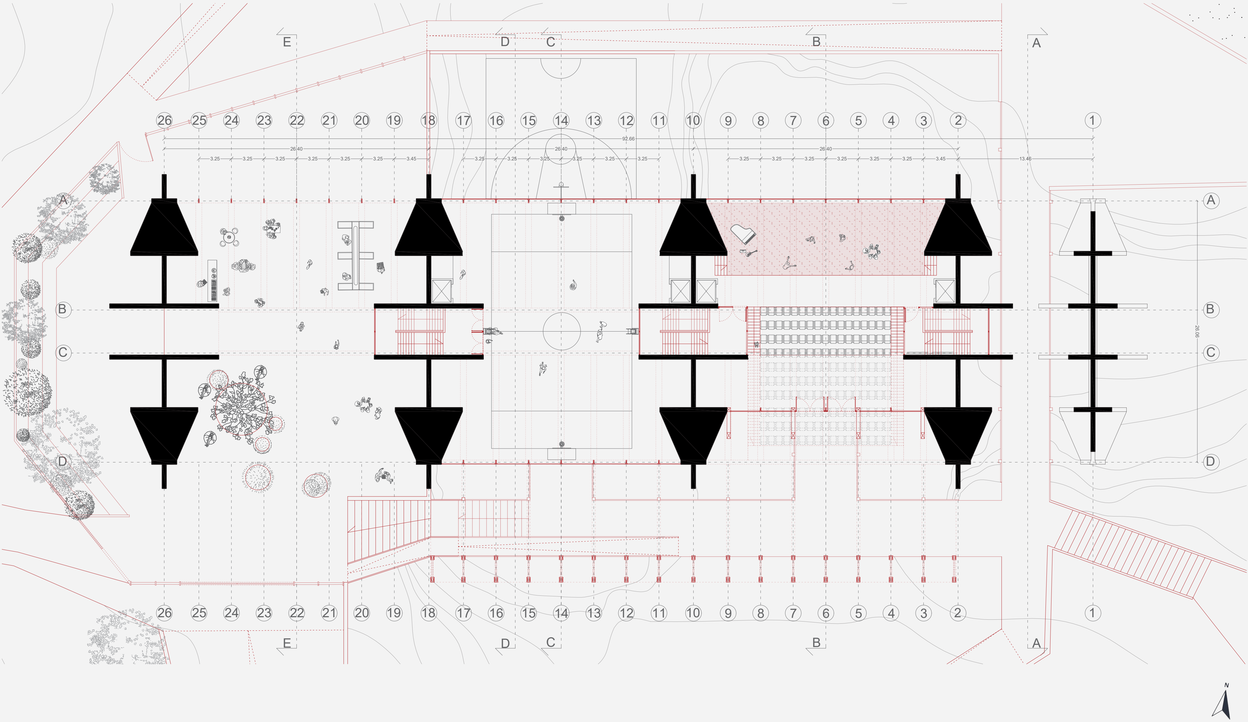
Planta Nivel 1 Escala 1/200
