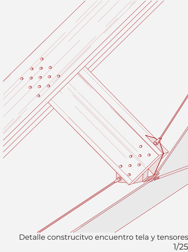
Detalle constructivo encuentro tela y tensores 1/25
