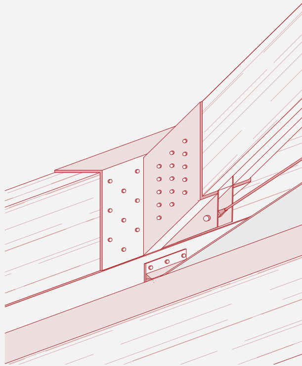
Detalle constructivo encuentro Cercha y viga 1/25
