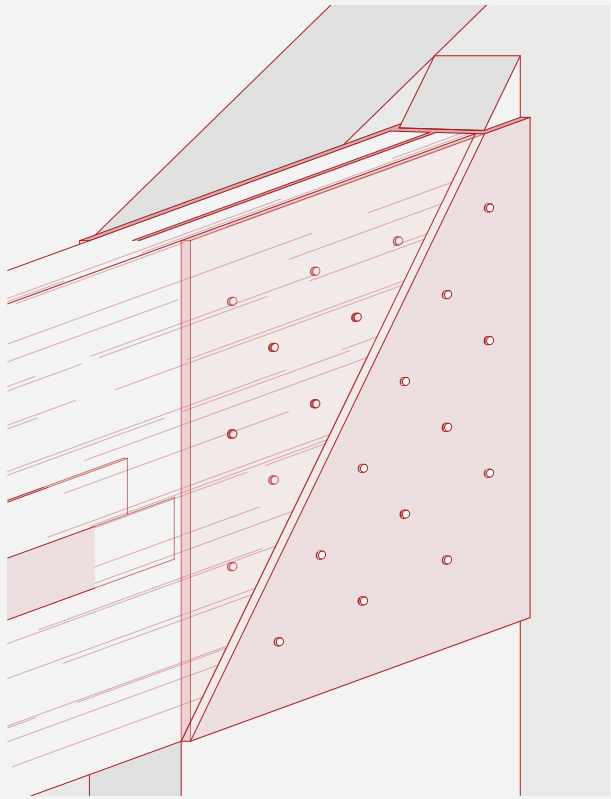
Detalle constructivo contrafuerte y viga 1/25
