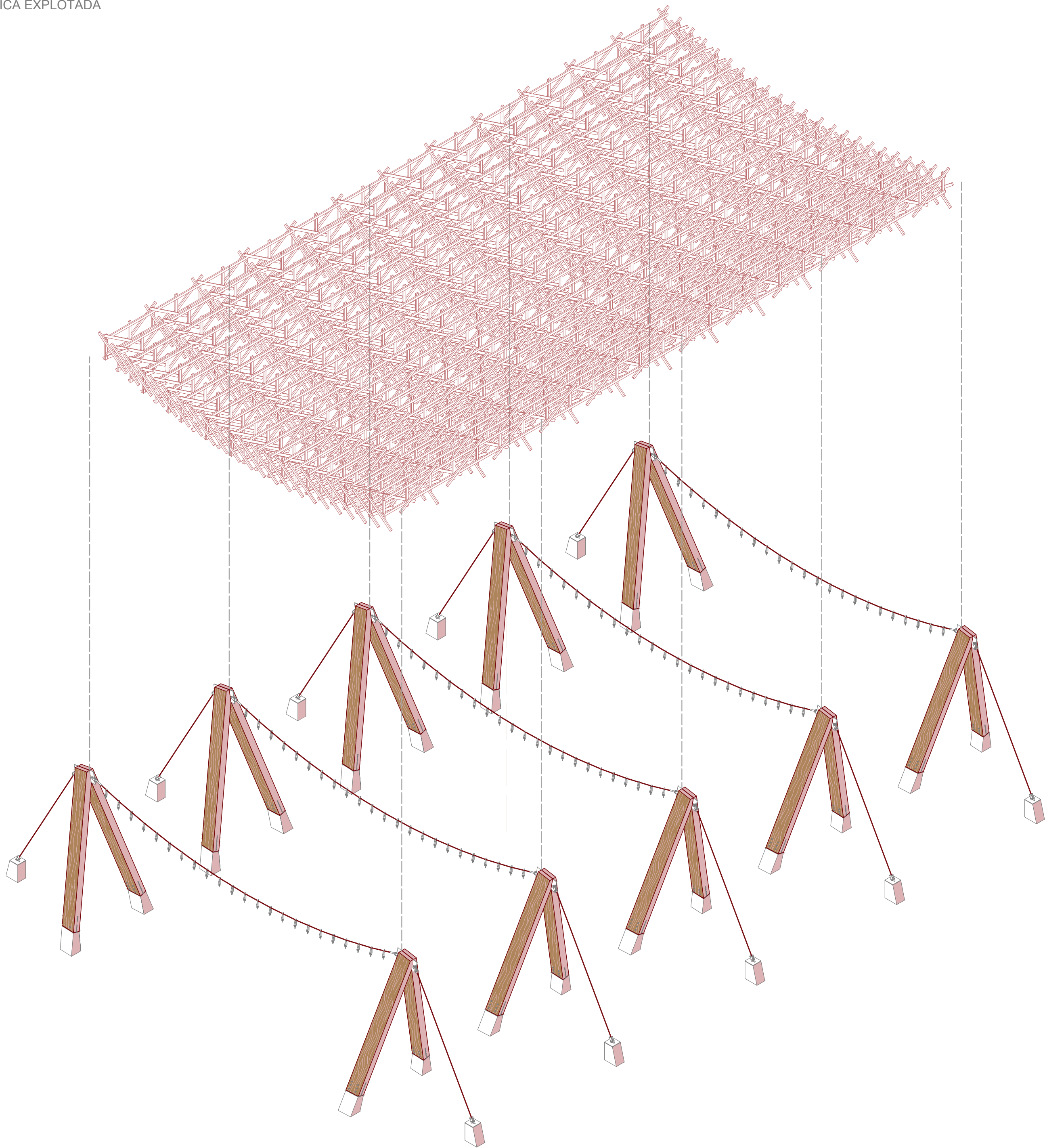
AXONOMÉTRICA EXPLOTADA
