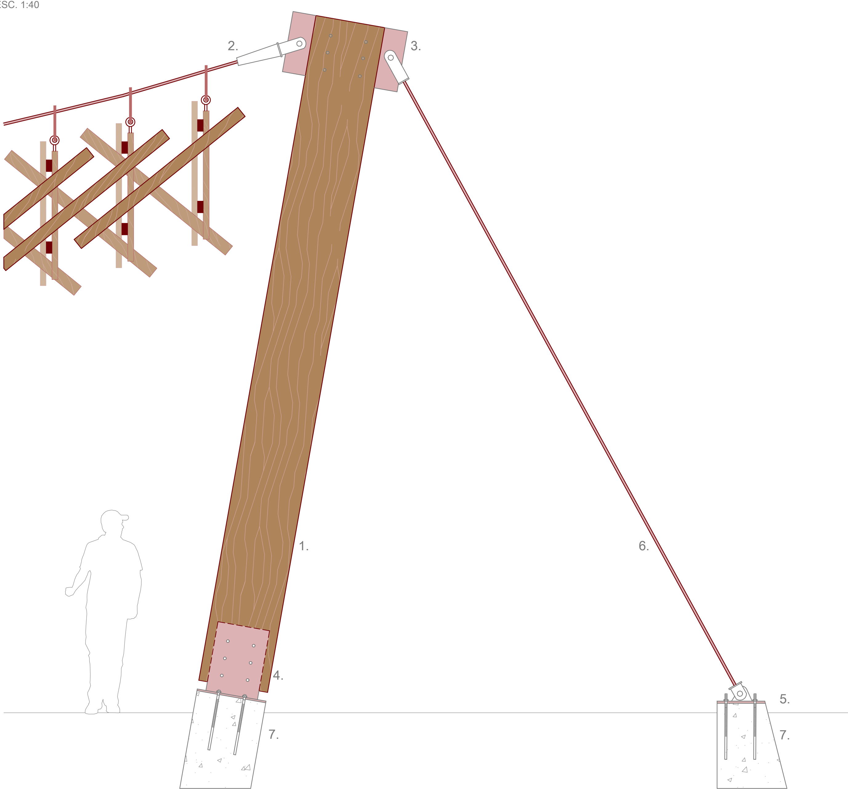
ESCANTILLÓN ESC. 1:40
