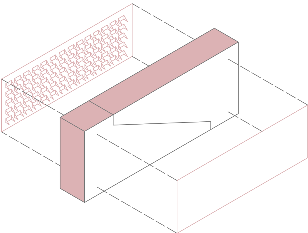
DETALLE ESC.1:20 EMPALME A TOPE CON PLACA DENTADA METÁLICA - 1MM 9X3 PULGADAS
