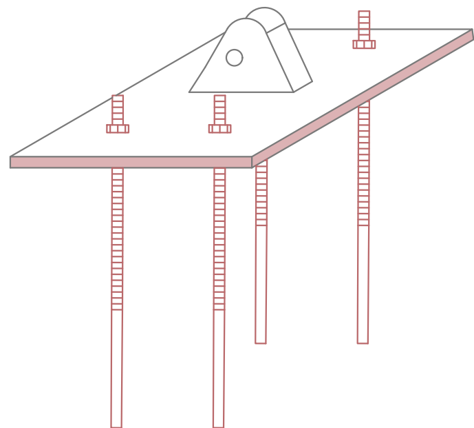
DETALLE ESC. 1:20 PLACA ANCLAJE TENSOR-BLOQUE HORMIGÓN, ACERO INOX. 50MM
