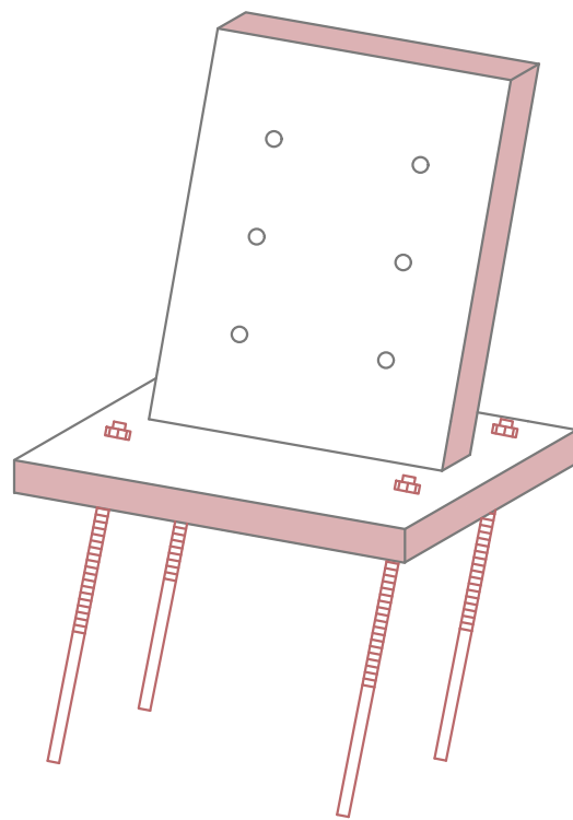
DETALLE ESC. 1:20 PLACA ANCLAJE PILAR-BLOQUE HORMIGÓN, ACERO INOX. 50MM
