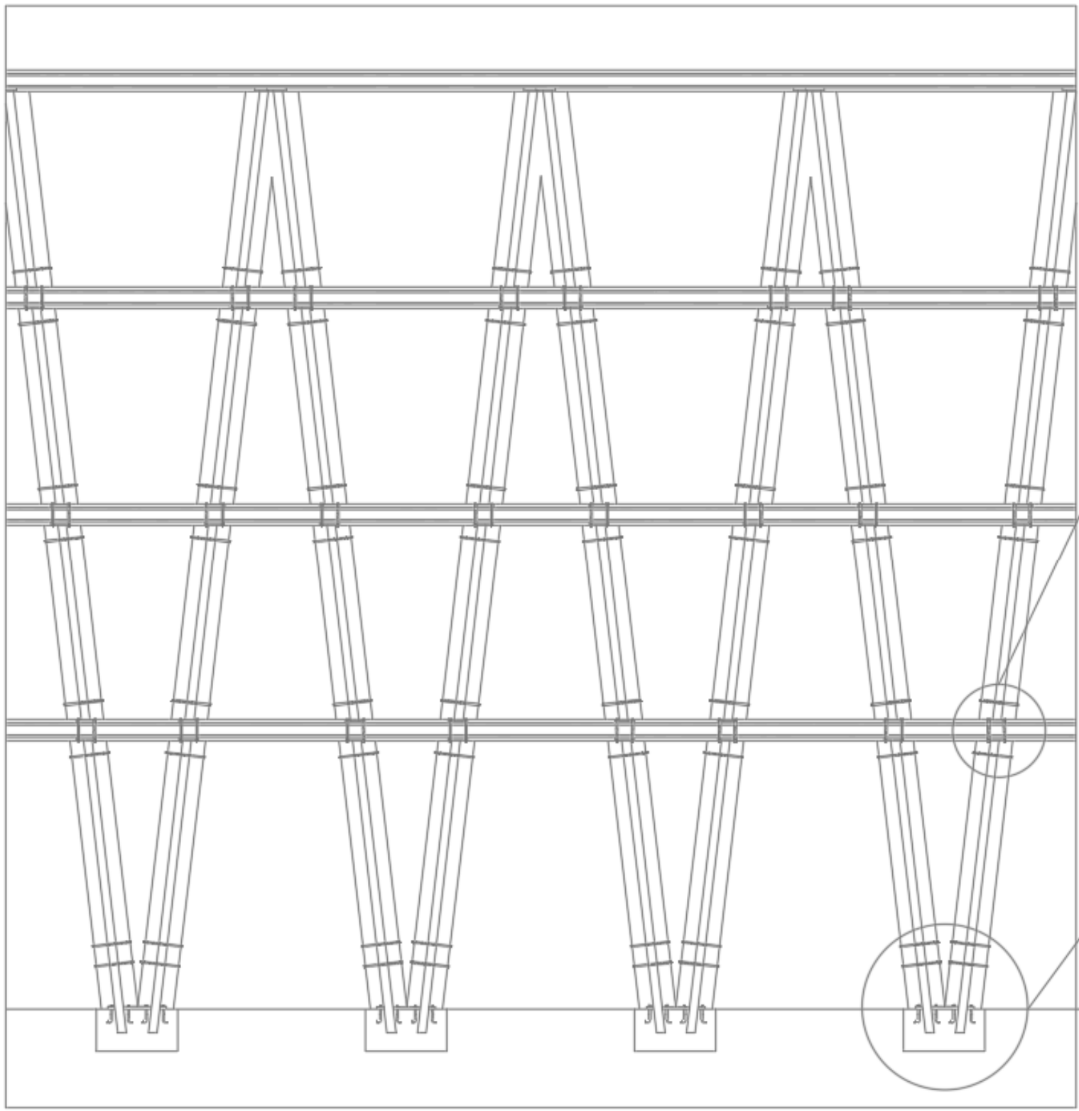
CORTE ESCANTILLON SOBRE ESTRUCTURA DE PILARES
