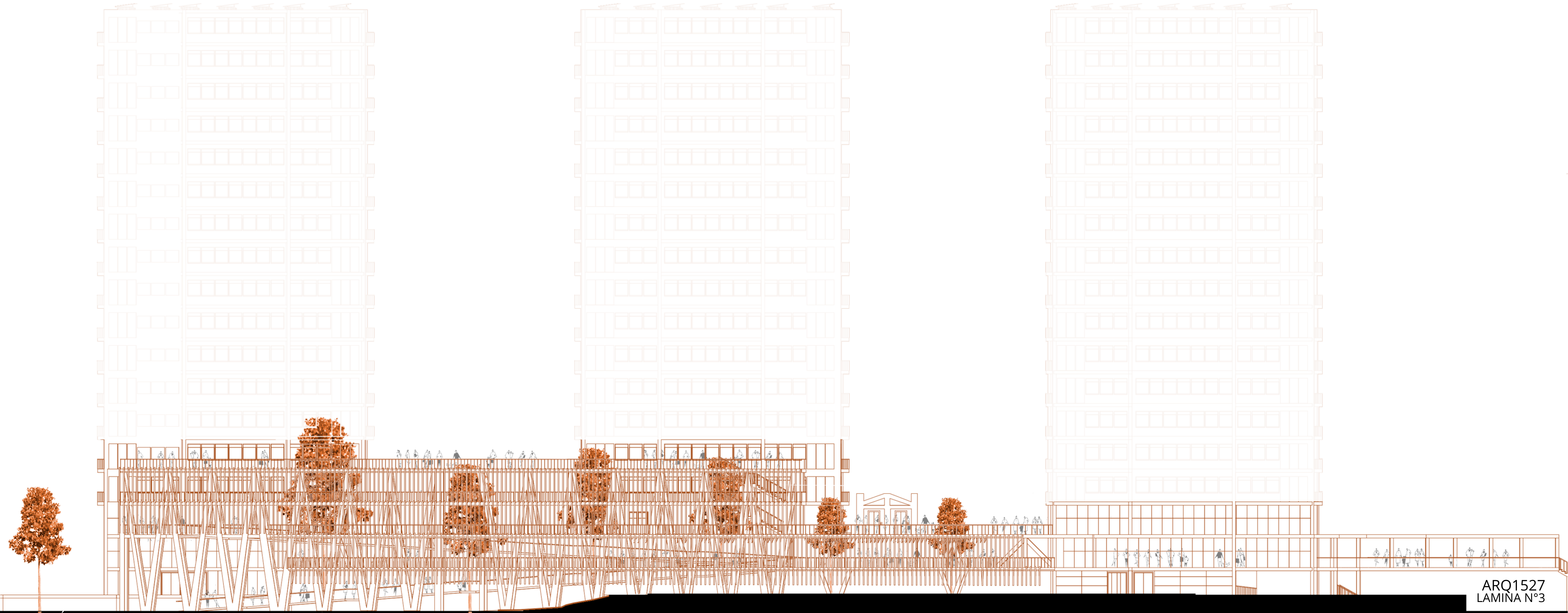
ELEVACIÓN ORIENTE ( CALLE JAIME EYZAGUIRRE )
