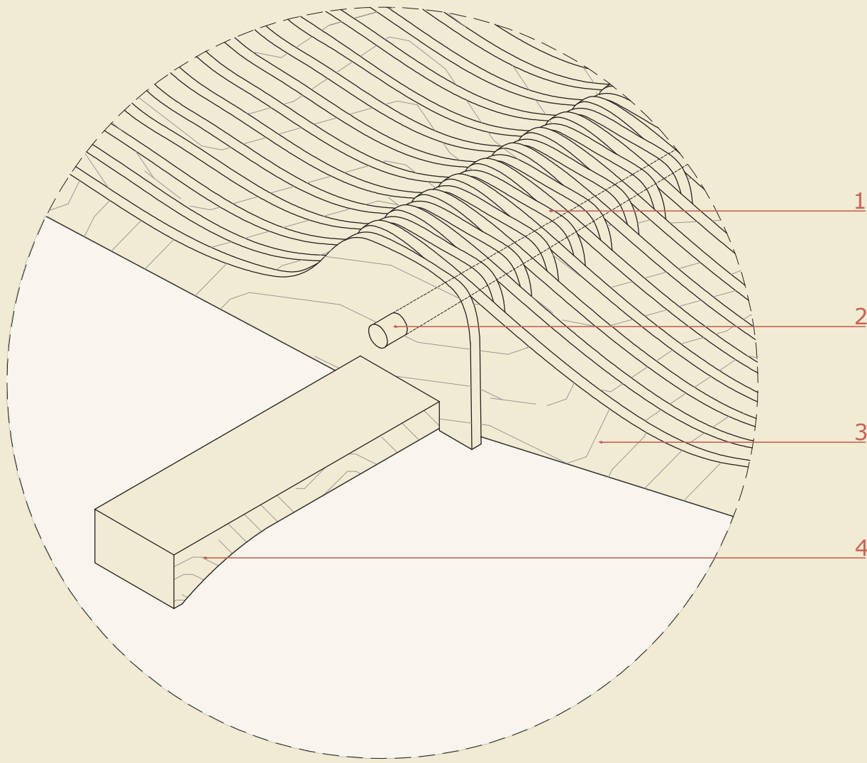
DETALLE 4 UNIÓN GRADA Y VIGA 1:10
