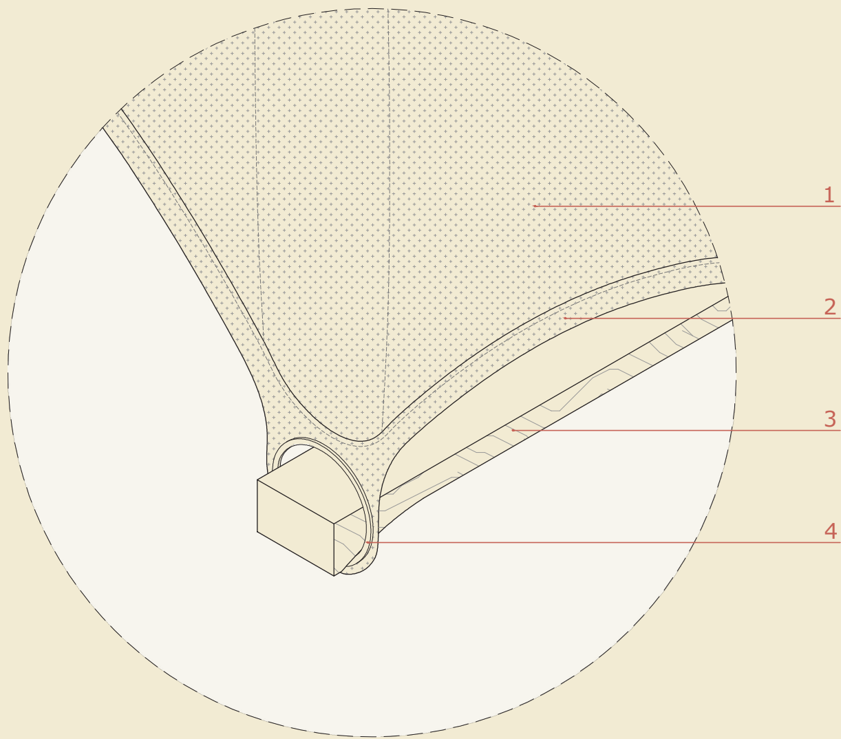
DETALLE 1 UNIÓN TELA Y VIGA 1:10
