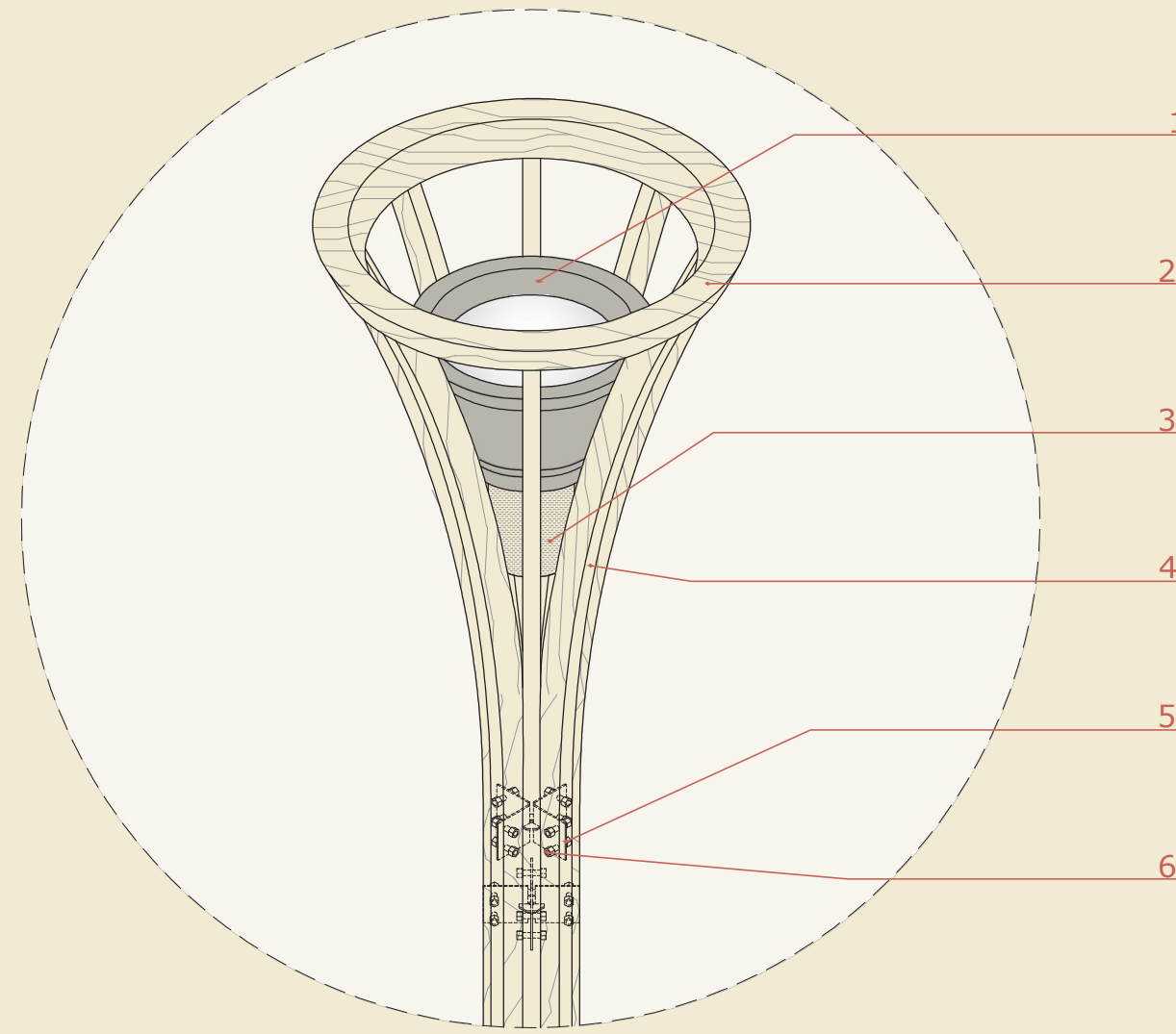
DETALLE 6 UNIÓN PILAR 1:10
