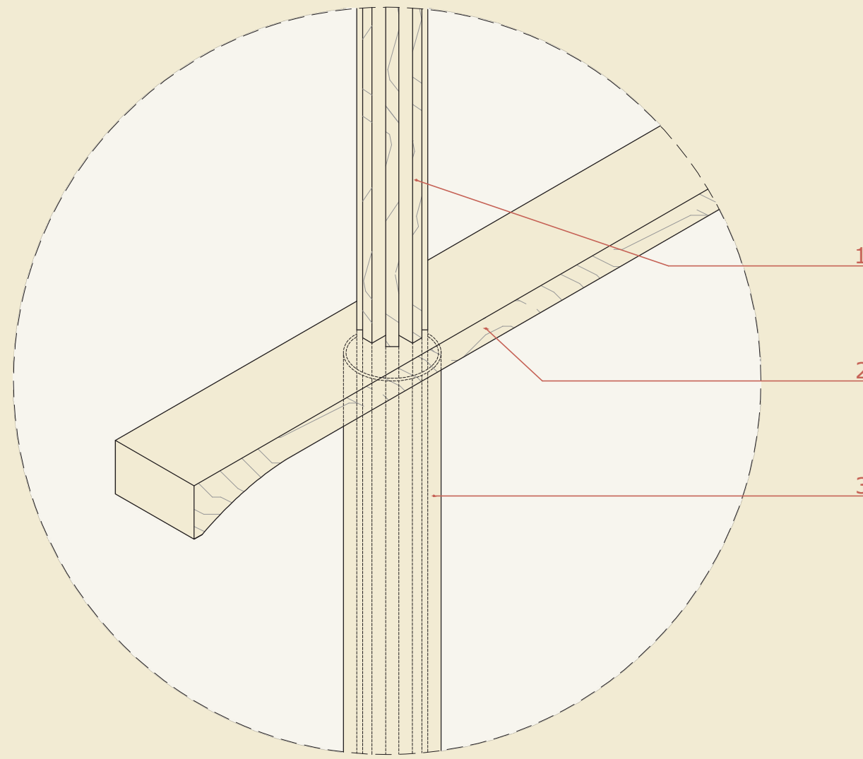
DETALLE 5 UNIÓN PILAR VIGA 1:10
