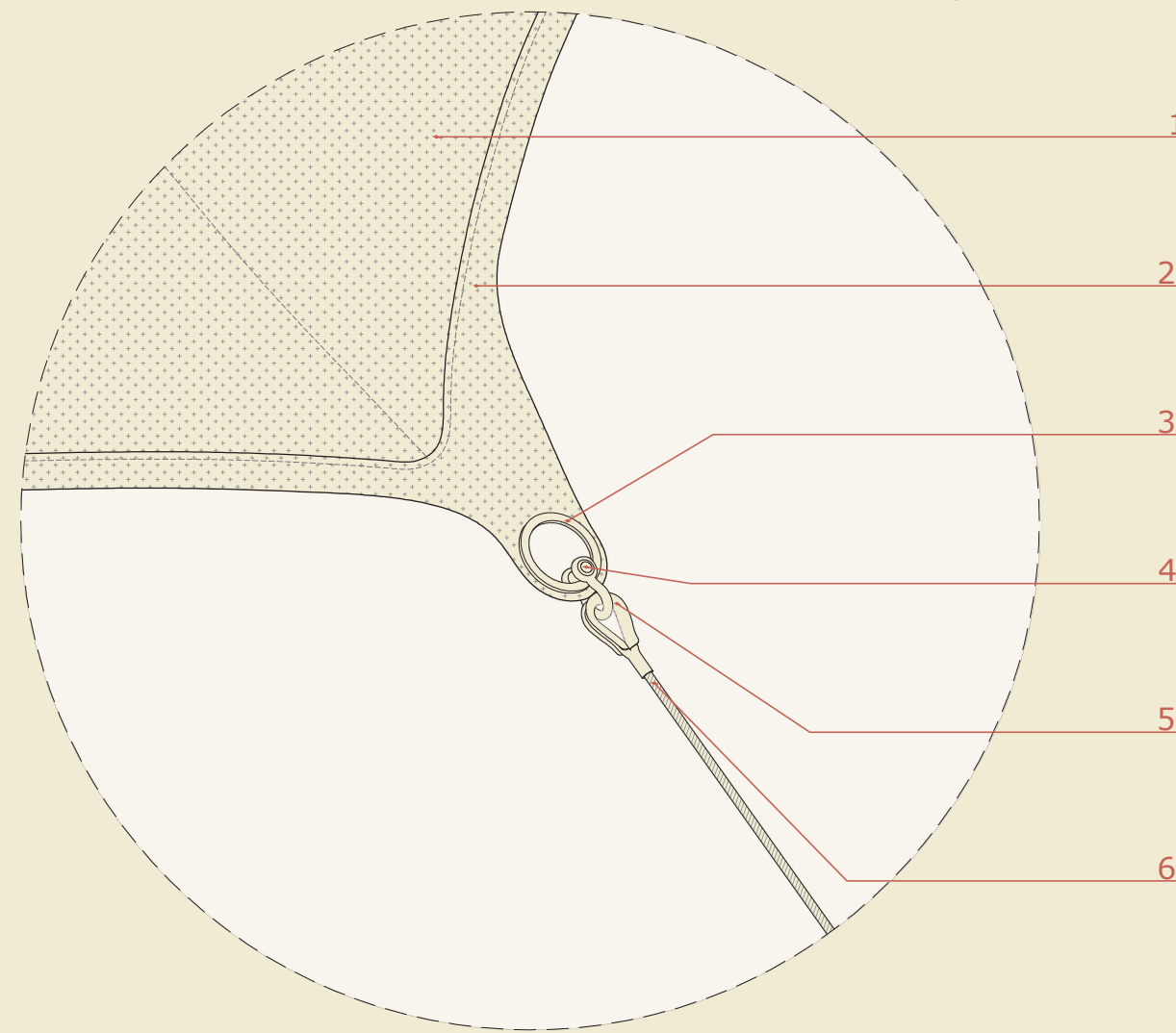
DETALLE 3 UNIÓN TELA Y CABLE 1:10
