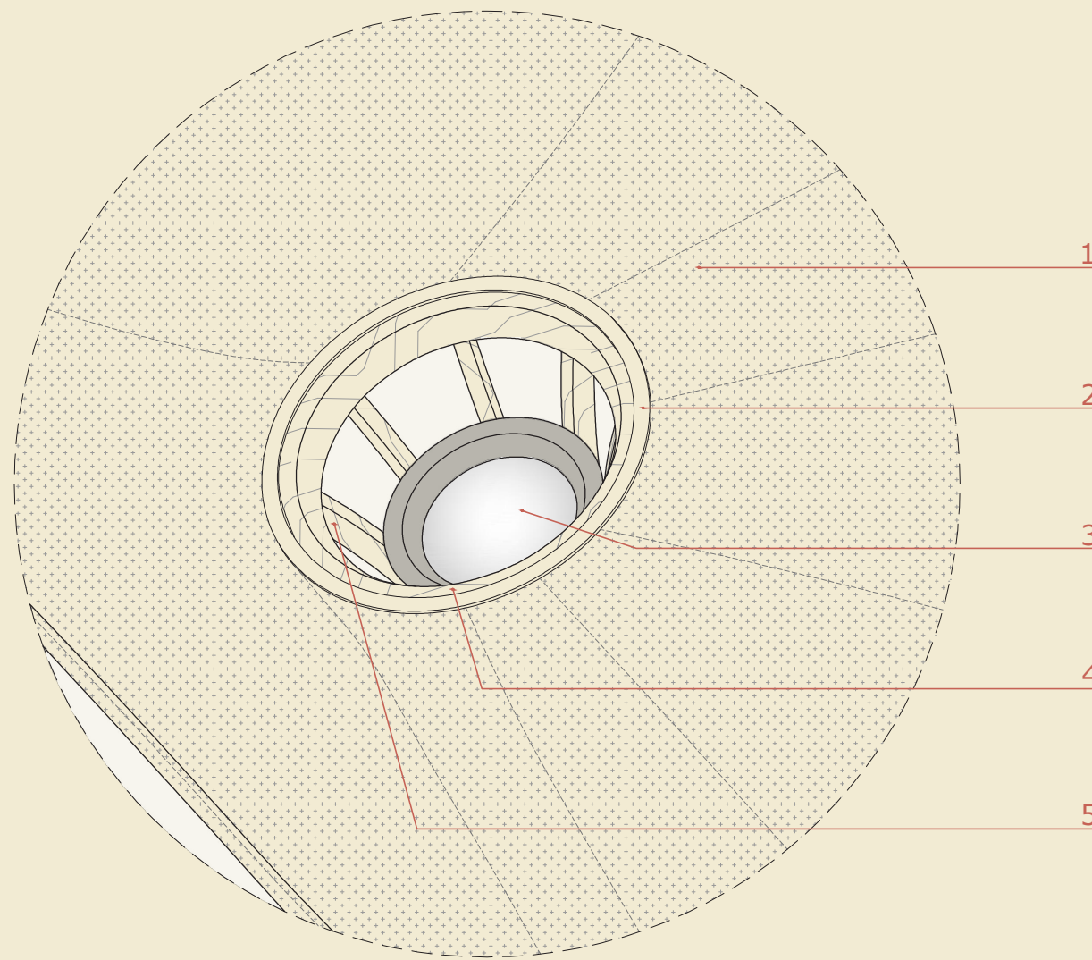
DETALLE 2 UNIÓN TELA Y PILAR 1:10
