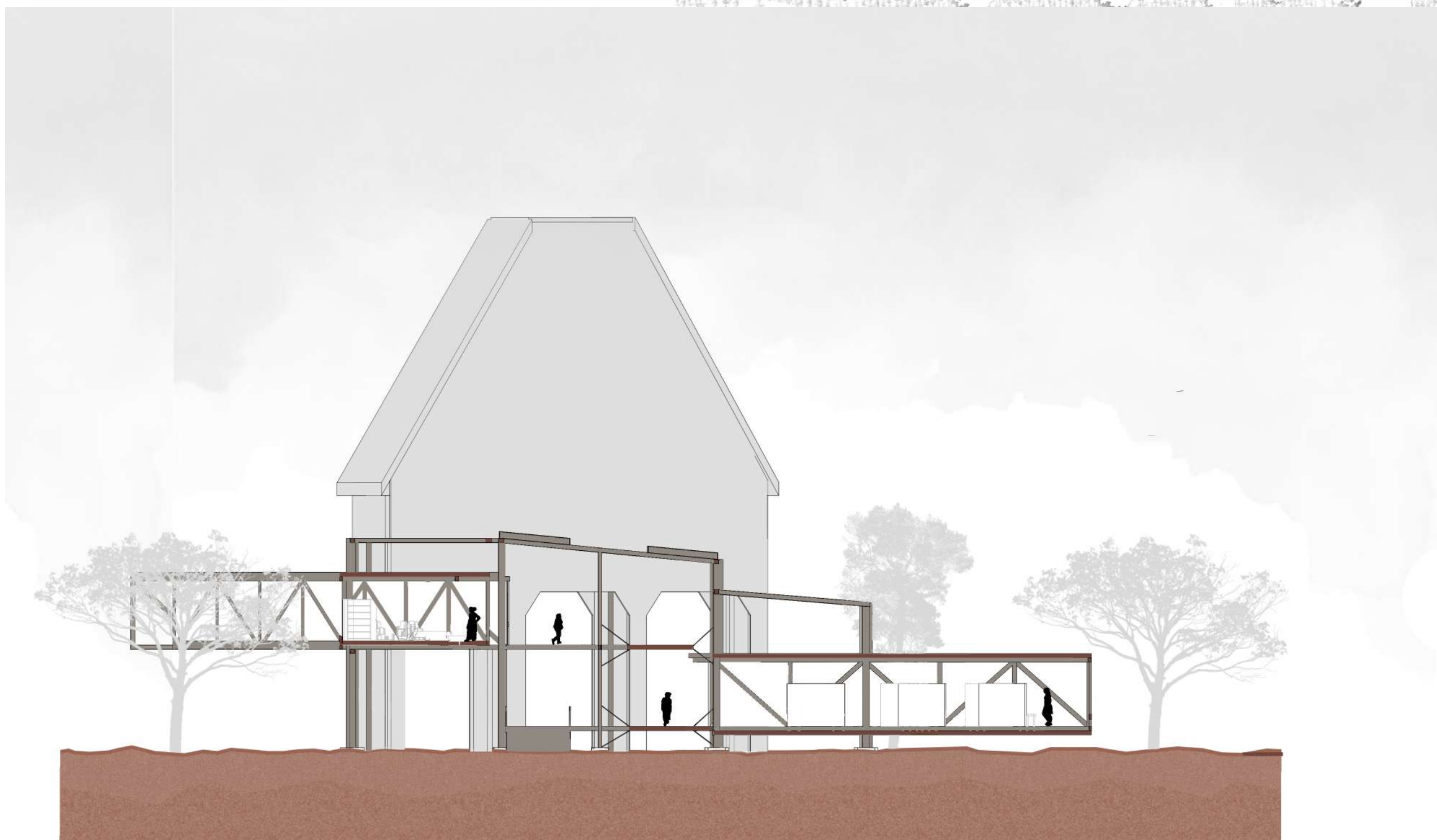
CORTE A-A' ESC. 1:200
