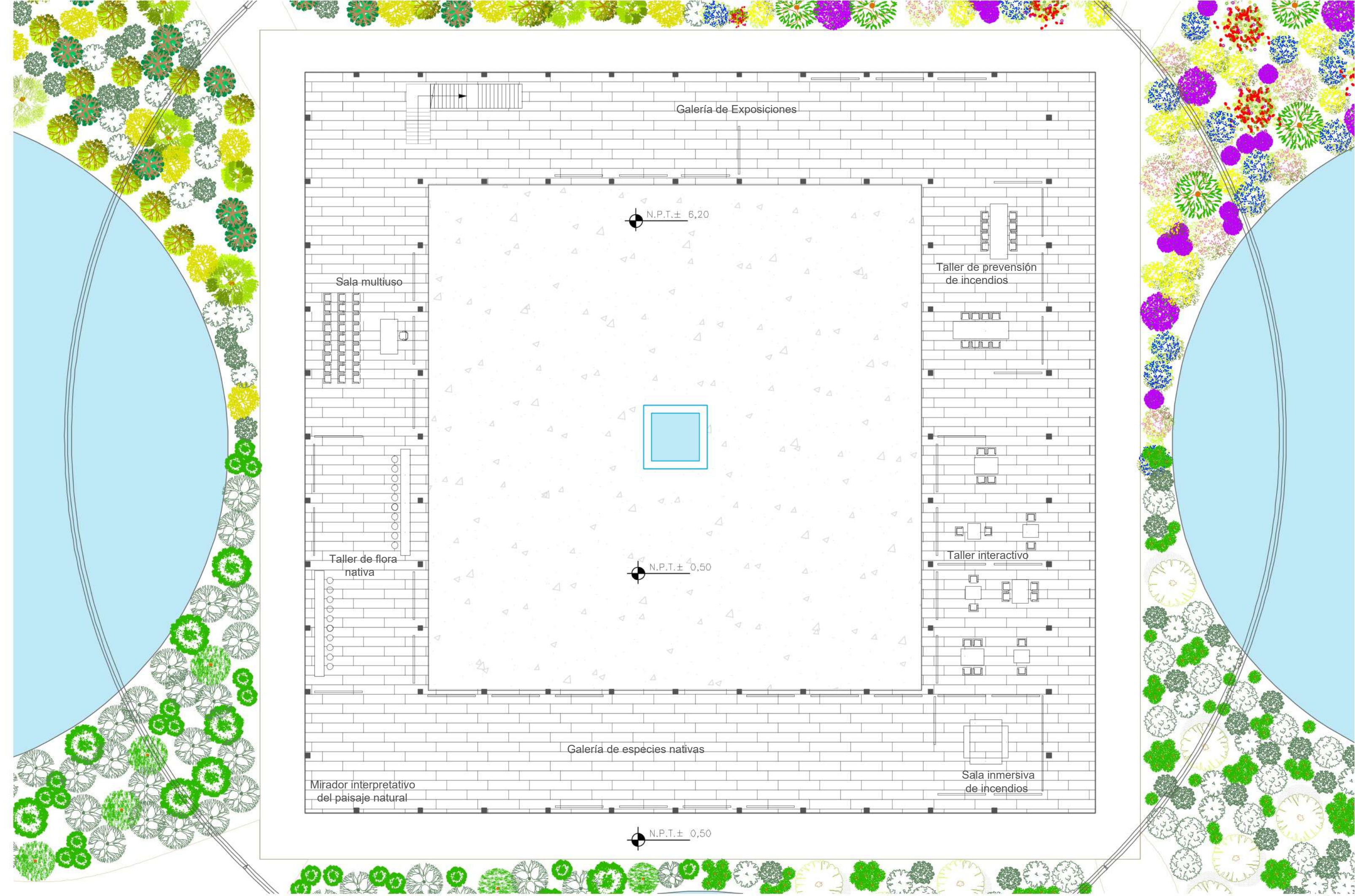
PLANTA NIVEL 2
