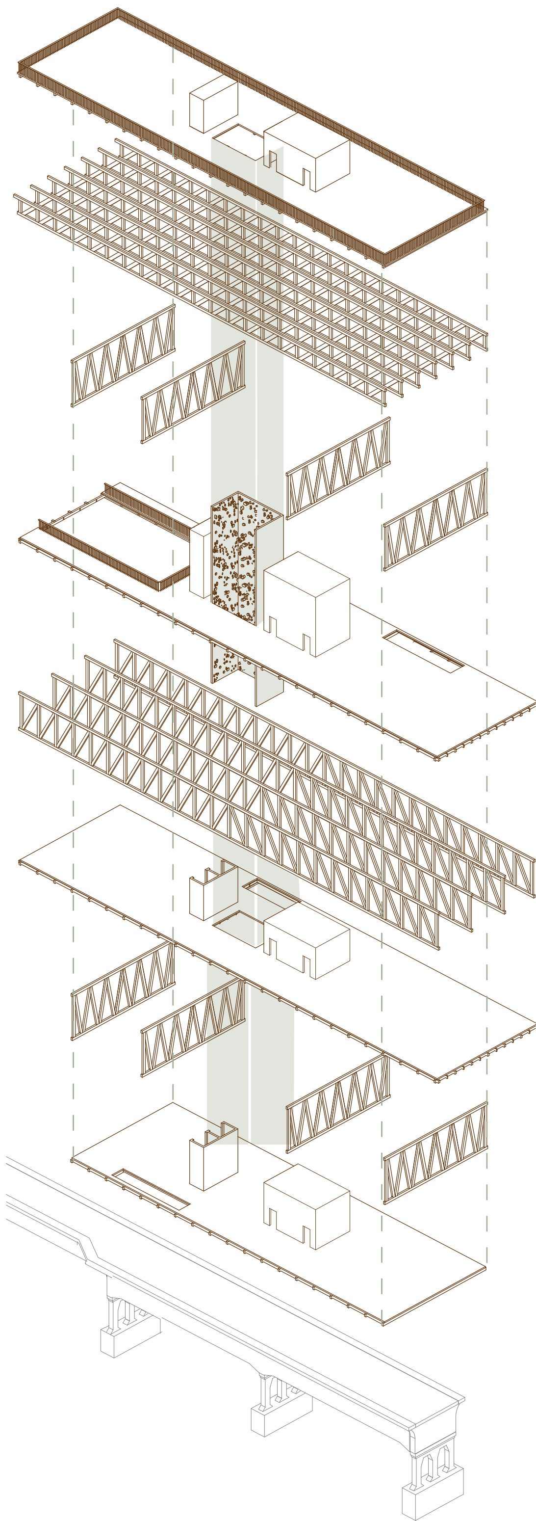
AXONOMÉTRICA EXPLOTADA
