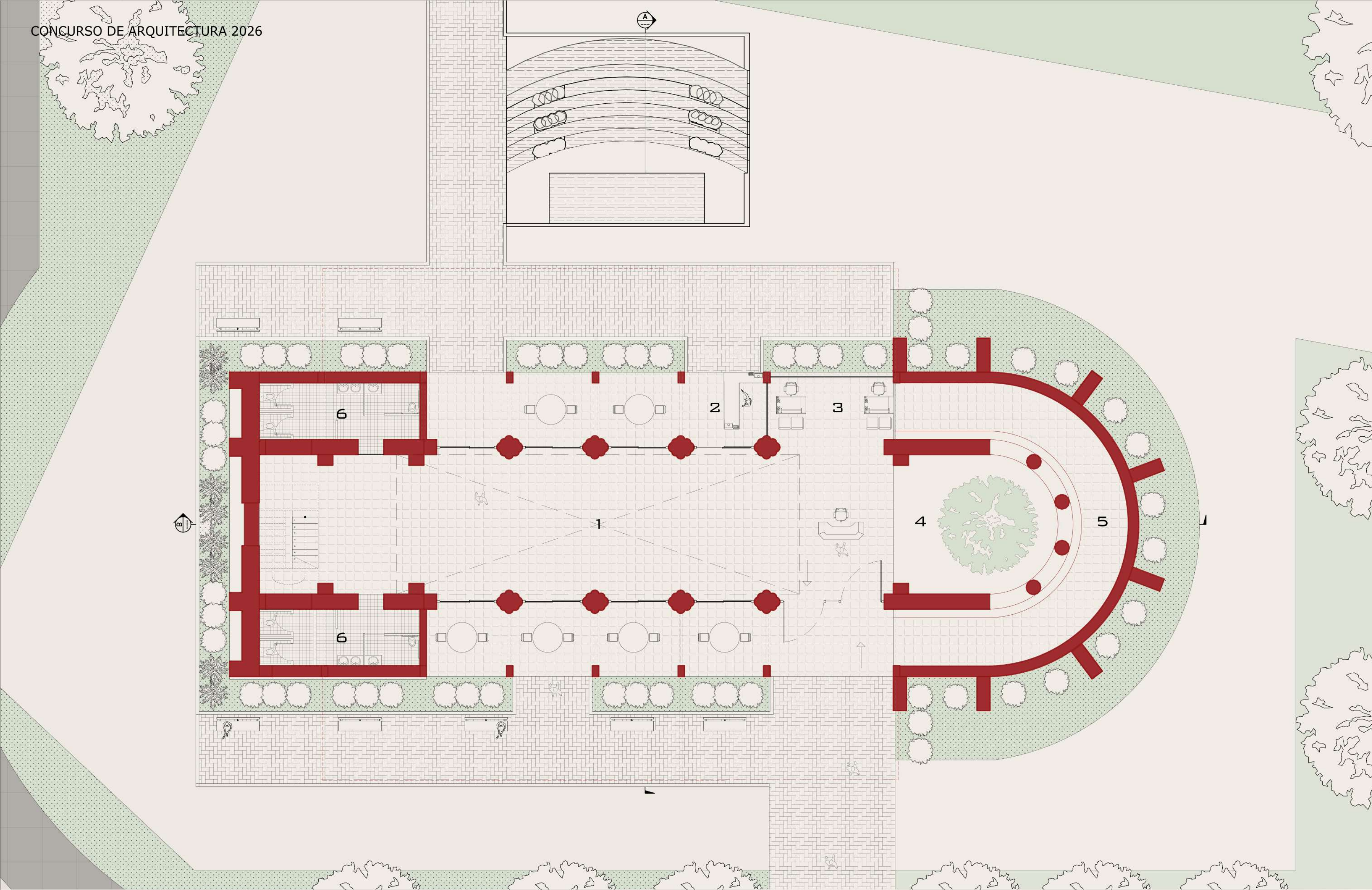
PLANTA 1º NIVEL Esc. 1:125
