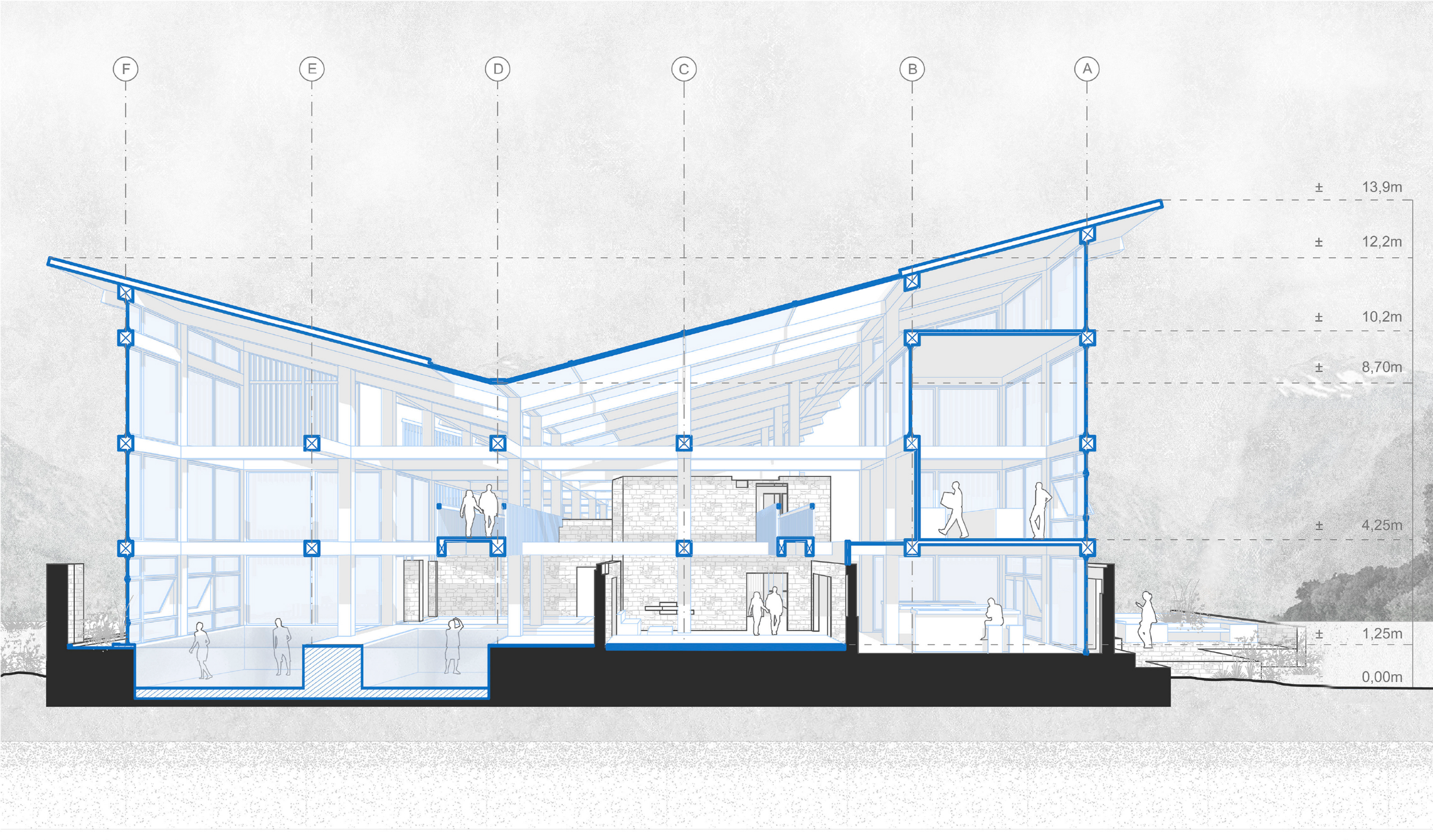
Corte transversal | escala 1:75
