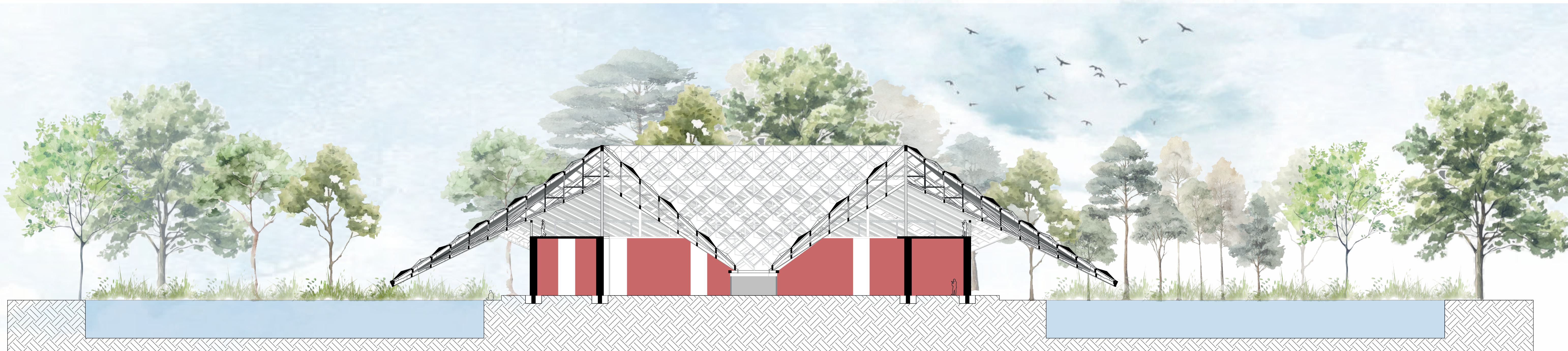
CORTE A-A' ESC. 1/200
