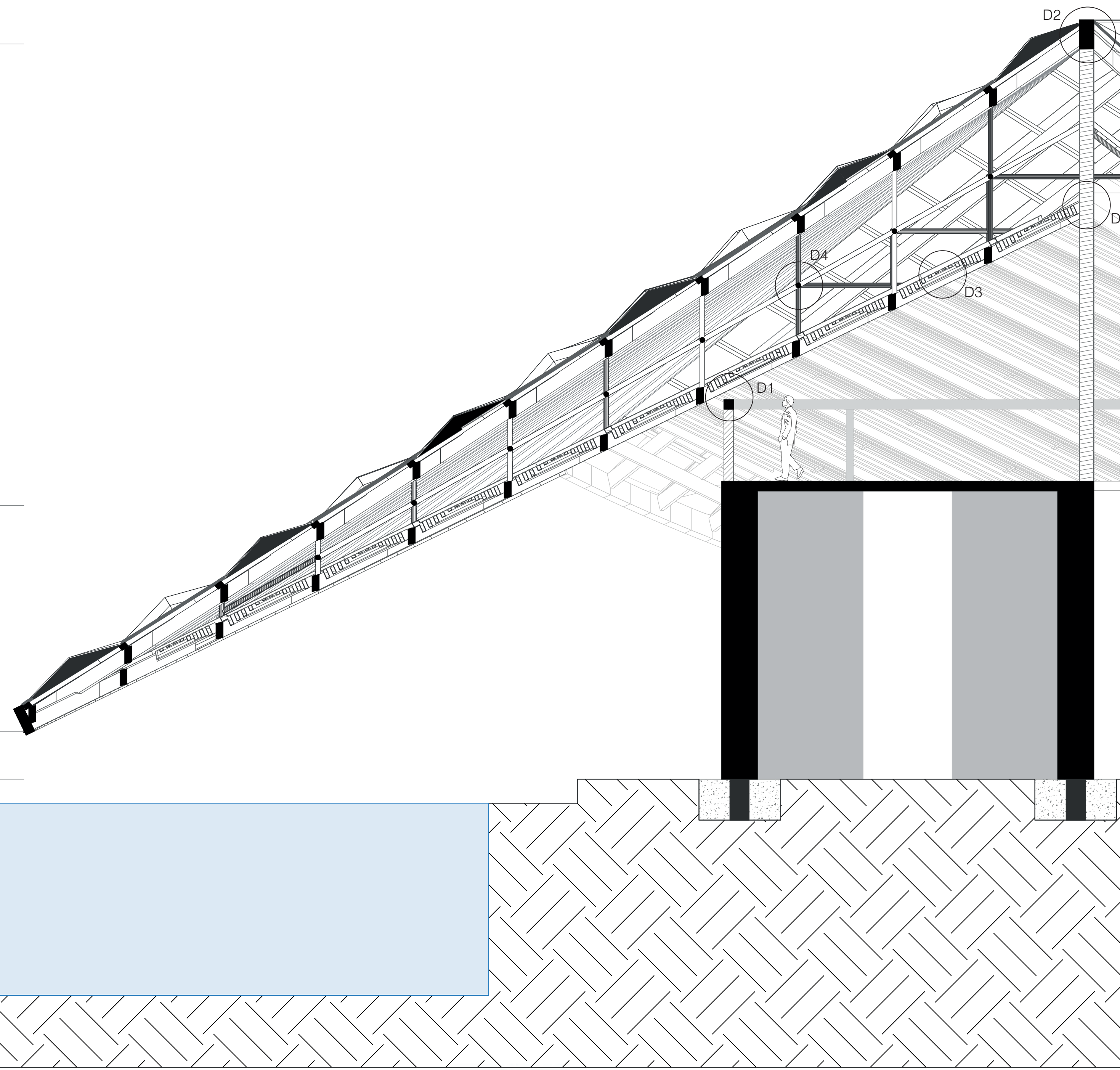
ESCANTILLON ESC. 1/60
