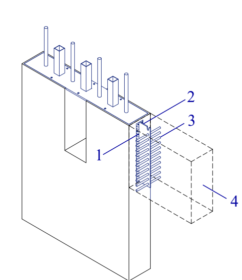
Nudo 3 | Esc. 1:25
