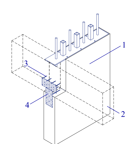
Nudo 2 | Esc. 1:25
