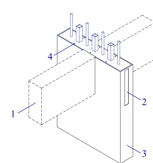
Nudo 1 | Esc. 1:25
