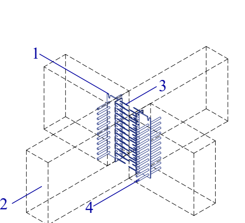
Nudo 4 | Esc. 1:25
