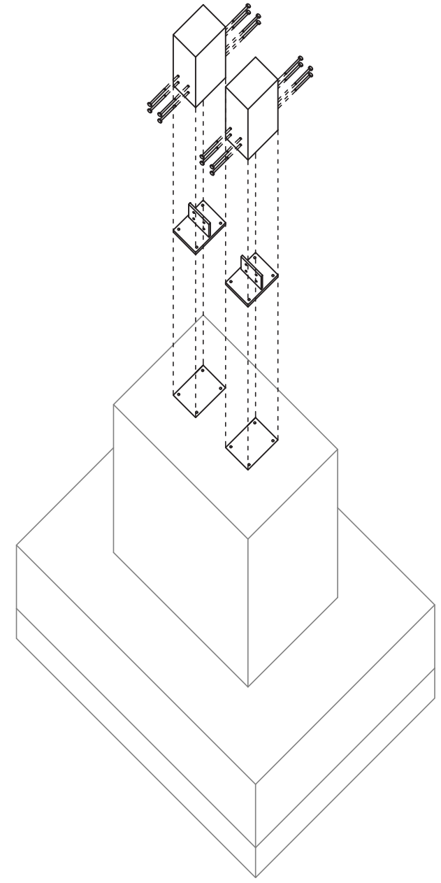
D2: Detalle conexión pasarela-tensor-pilar
