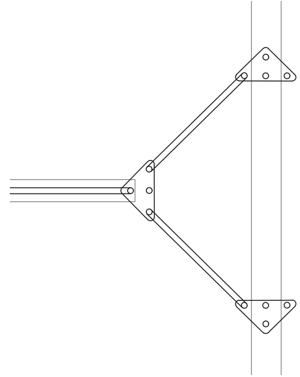
D2: Detalle conexión pasarela-tensor-pilar
