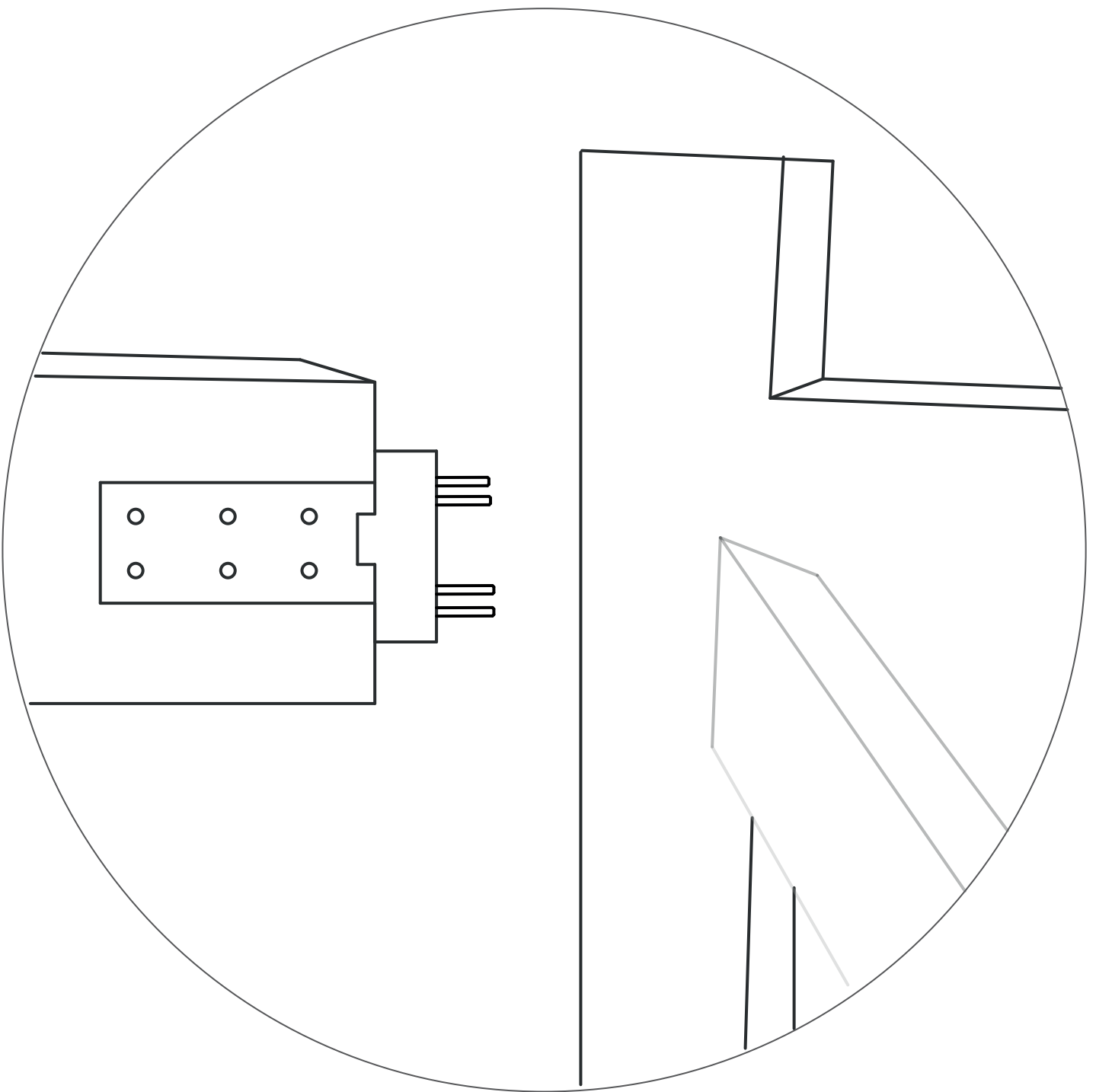
DETALLE 5
