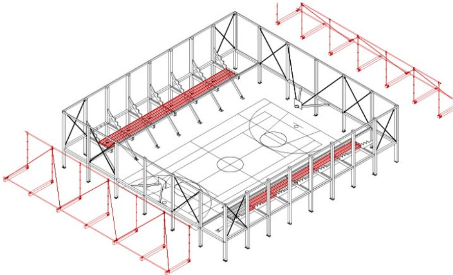
5. MONTAJE DE DE ESTRUCTURAS METÁLICAS: ESCALERAS Y GRADERÍAS
