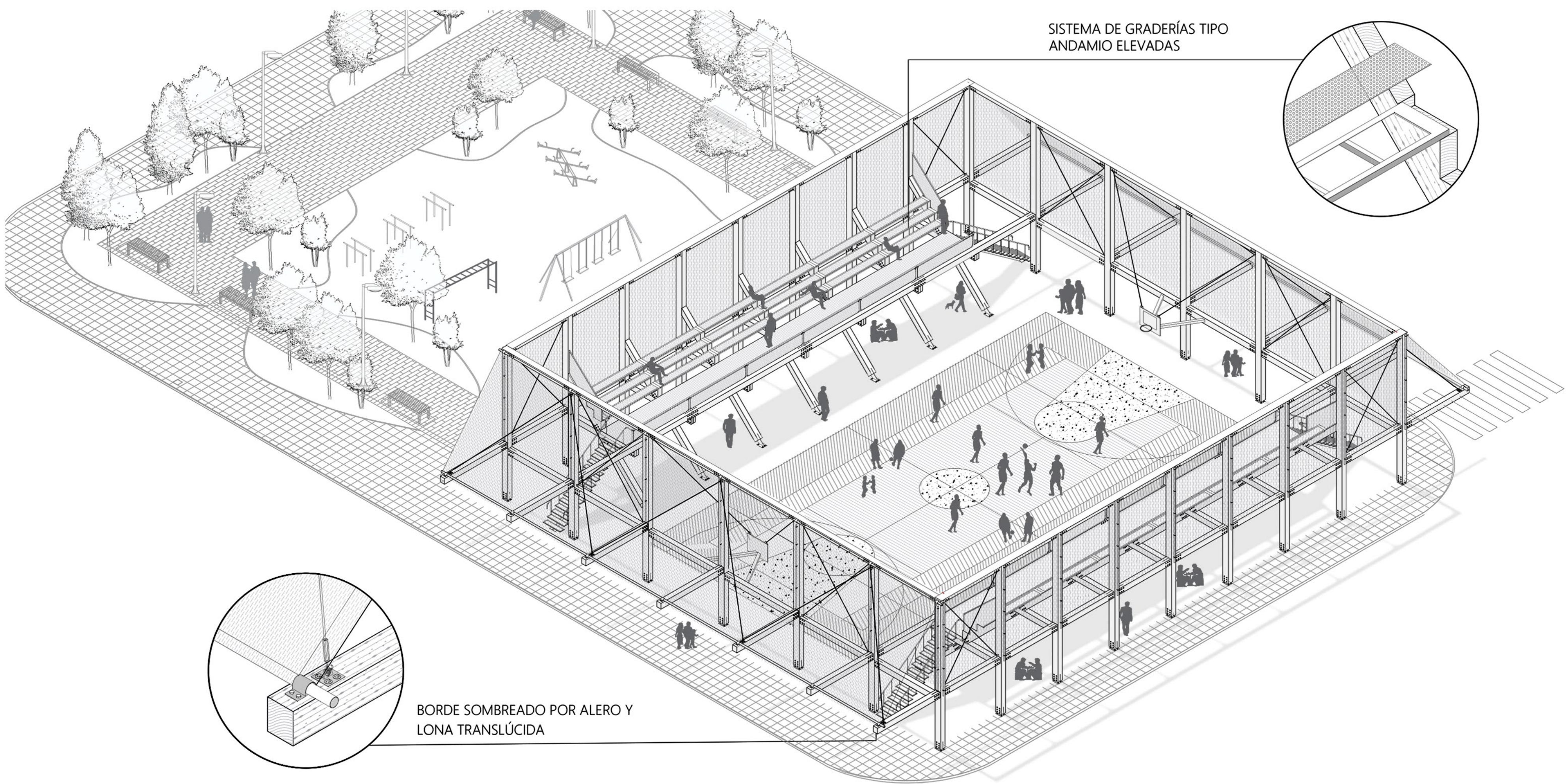
AXONOMÉTRICA FUNCIONAMIENTO (1:150)
