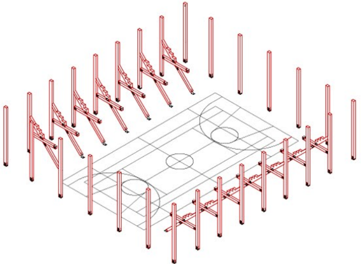
3. VIGAS DE AMARRE Y TENSORES
