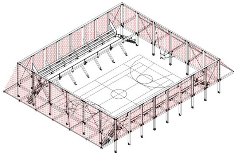
SECUENCIA DE ARMADO (1:500)
