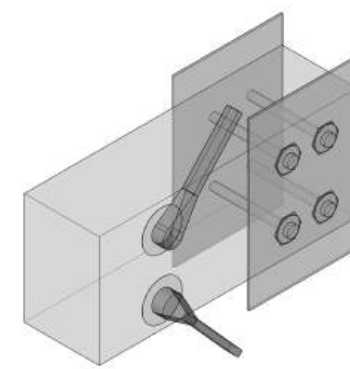
DETALLE 3 ANCLAJE TENSOR DOBLE
