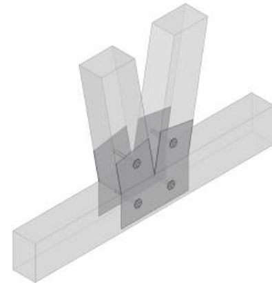
DETALLE 2 UNIÓN DE MADERA CON HERRAJE METÁLICO
