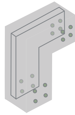
DETALLE 1 UNIÓN ESTRUCTURAL CODO
