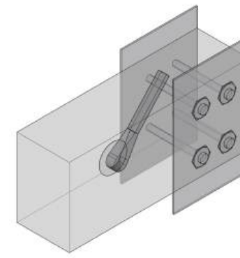
DETALLE 4 ANCLAJE TENSOR
