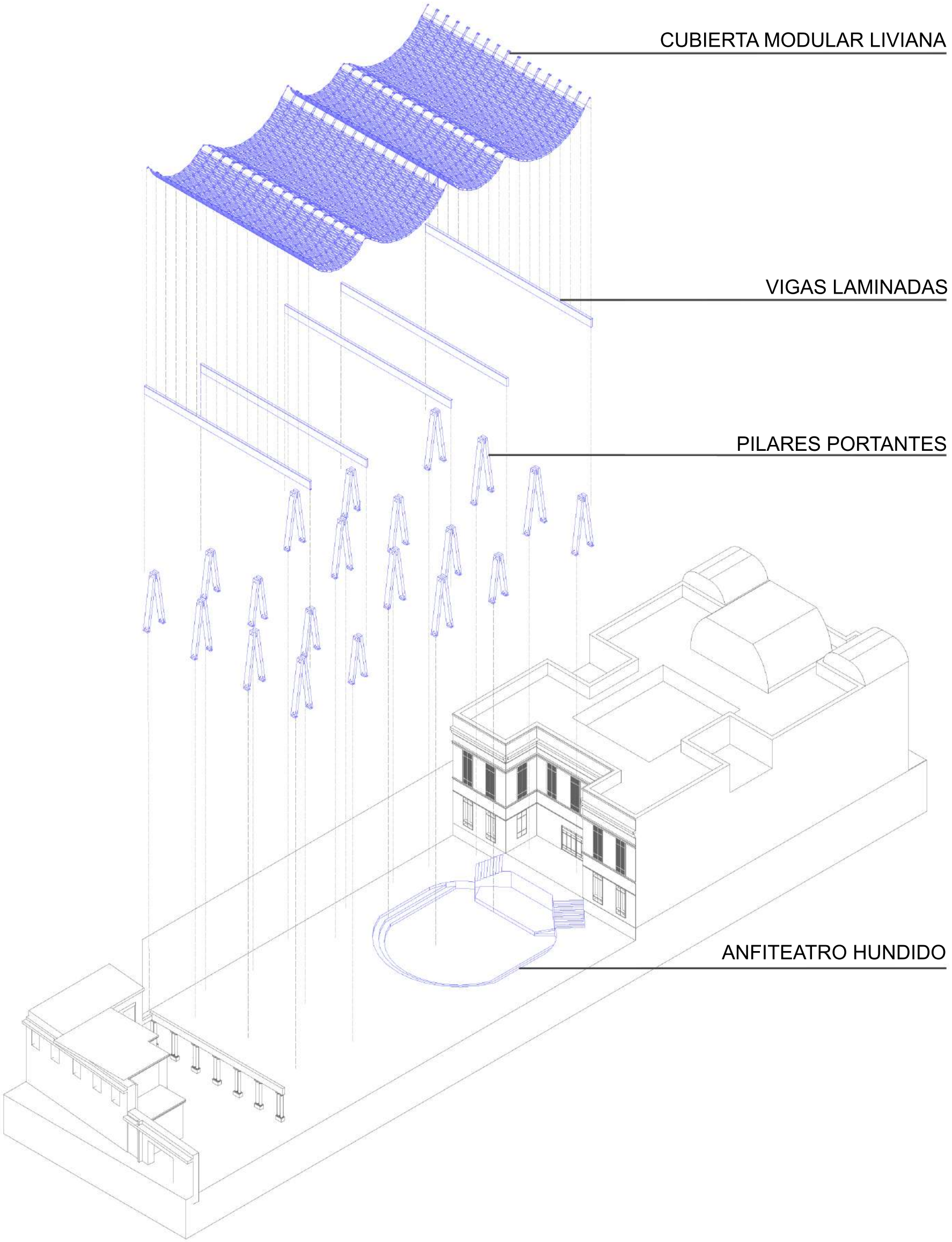
ISOMÉTRICA EXPLOTADA
