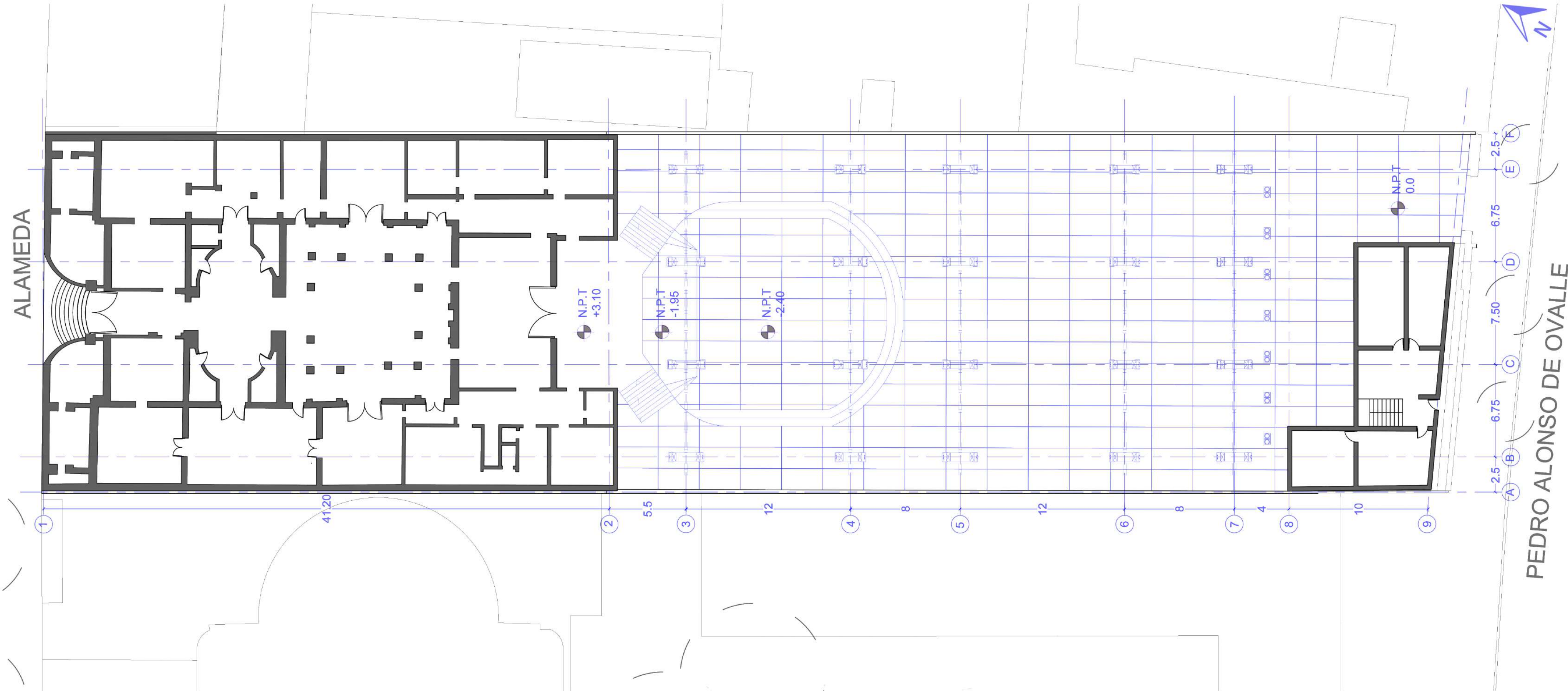
PLANO SUELO 1: 200
