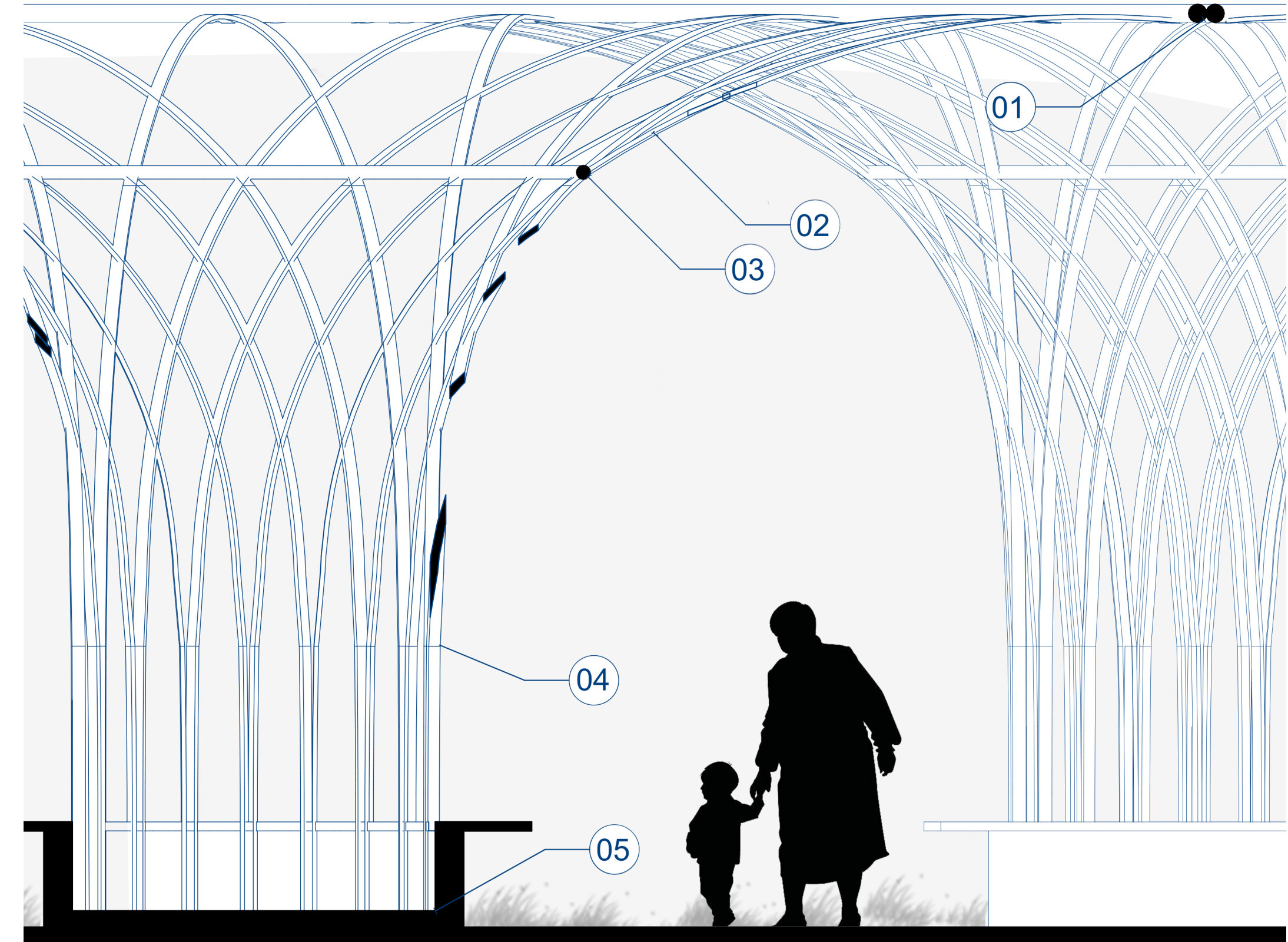
CORTE - DETALLE CONSTRUCTIVO ESC: 1 / 25
