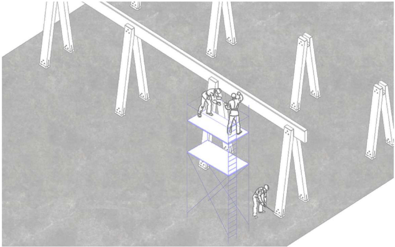
3. CONSTRUCCIÓN DE ESTRUCTURA
