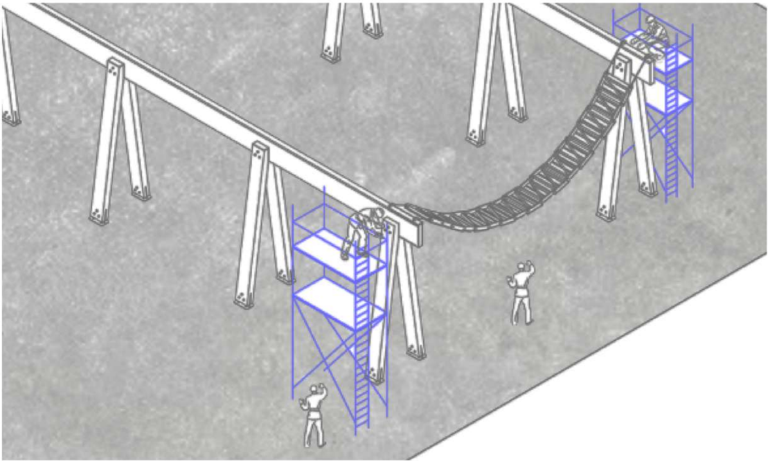
4. INSTALACIÓN DE MODULOS DE MADERA
