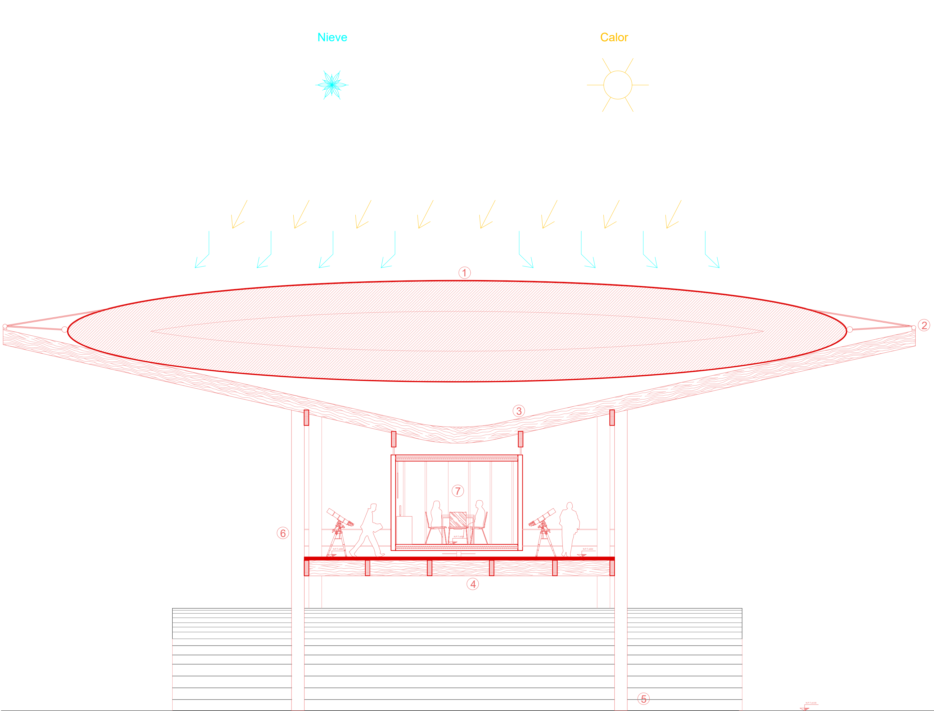
Corte C - C' ESC: 1:75
