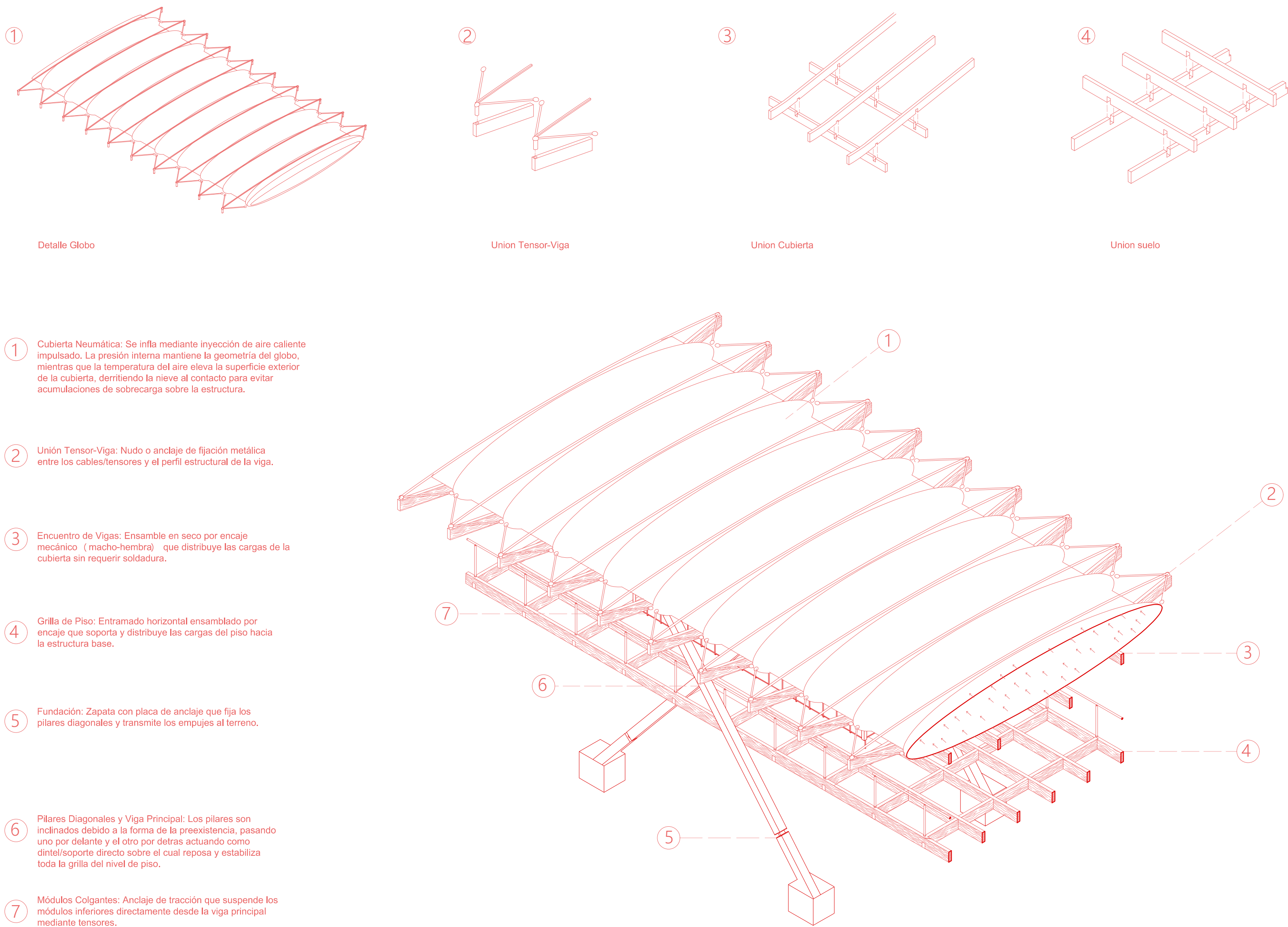
Isometrica Modulo ESC: 1:250
