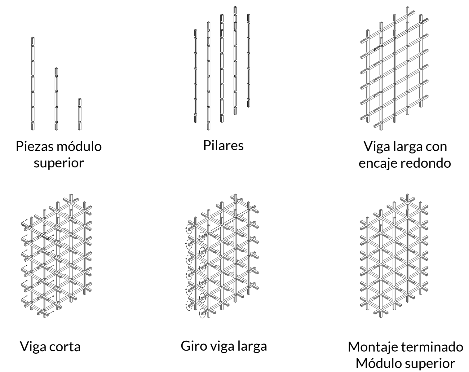
Sistema de Anclaje Japonés de tres piezas
