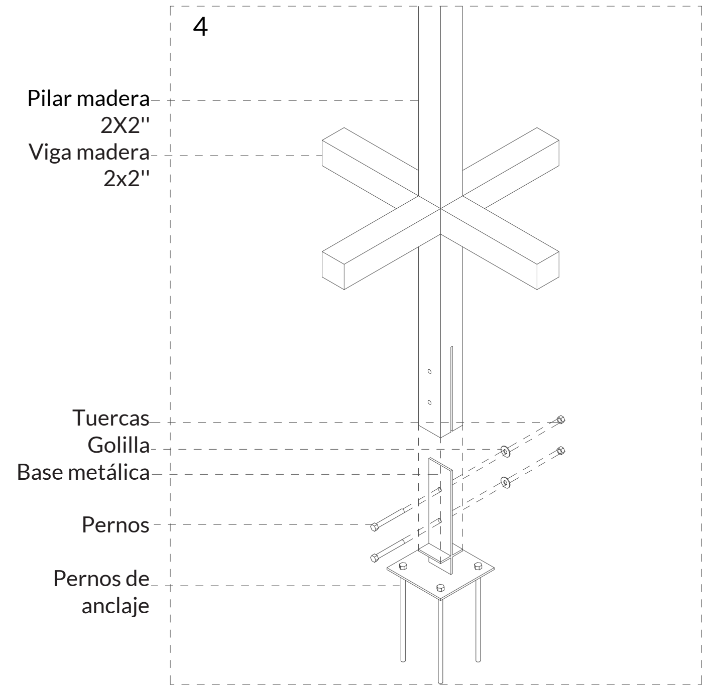
Sistema de Anclaje Japonés de tres piezas
