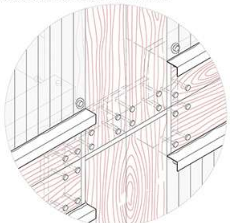
Detalle cosntructivo 2: union estructura
