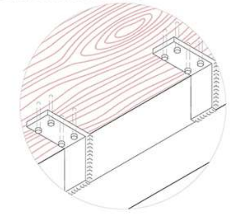
Detalle cosntructivo 4: union CLT
