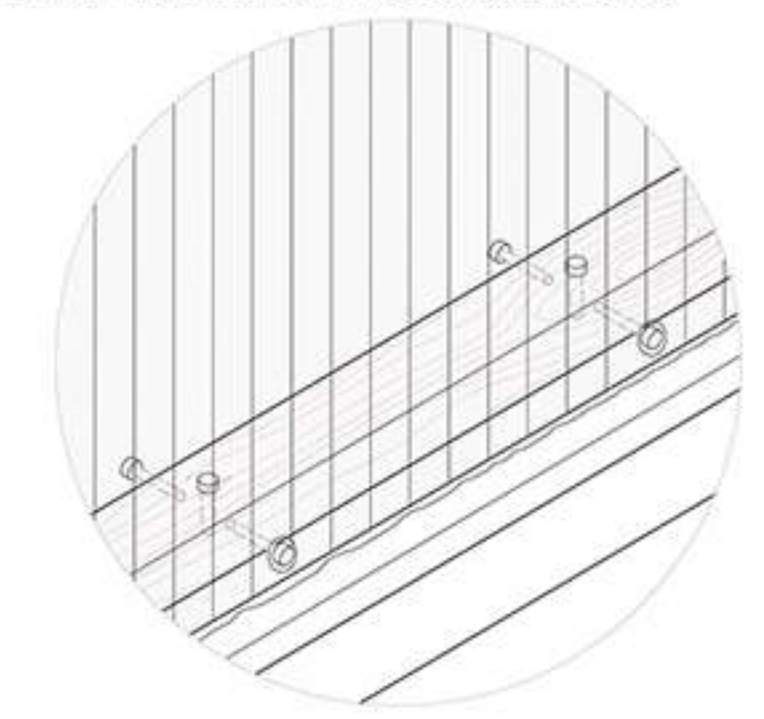
Detalle cosntructivo 3: marcos de policarbonato
