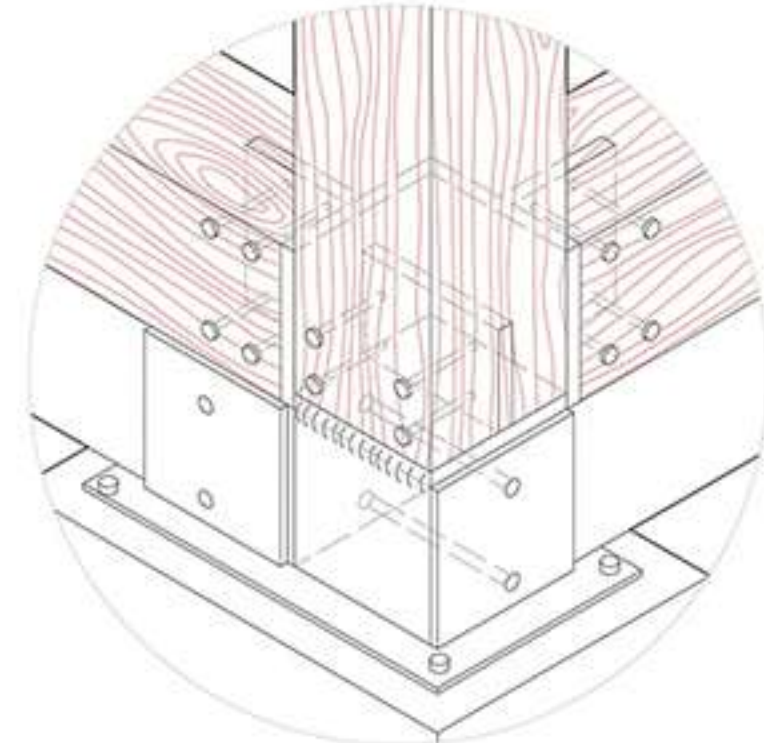
Detalle cosntructivo 5: union estructura a suelo
