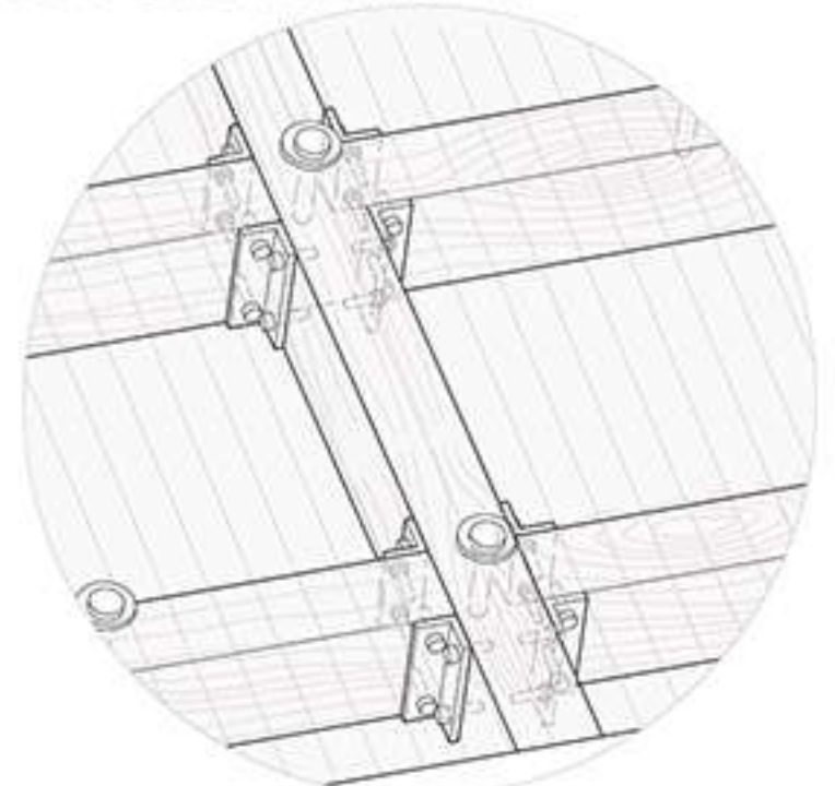
Detalle cosntructivo 1: techumbre
