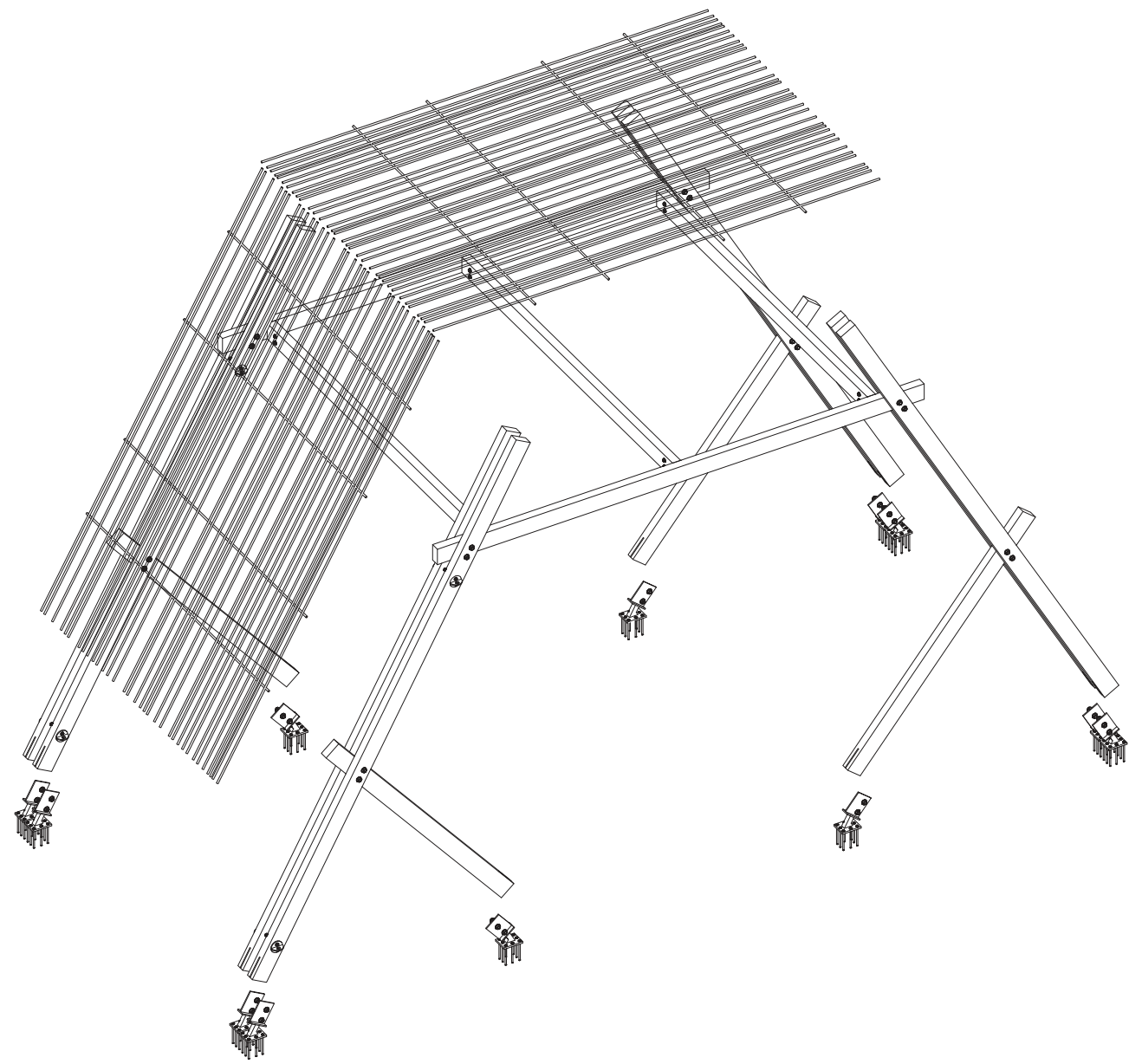
DETALLE ESTRUCTURA ESC. 1:25
