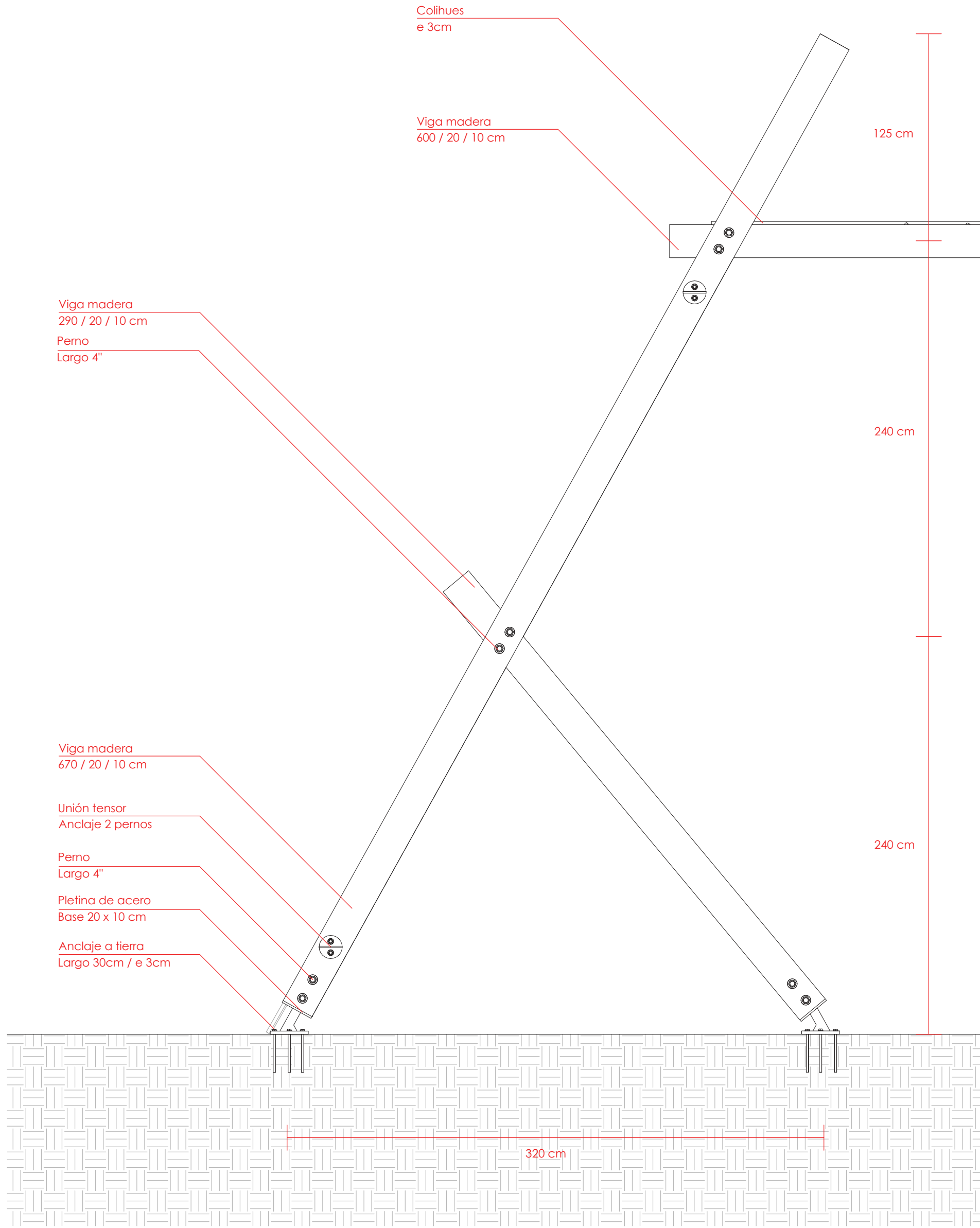
DETALLE ESTRUCTURA ESC. 1:25
