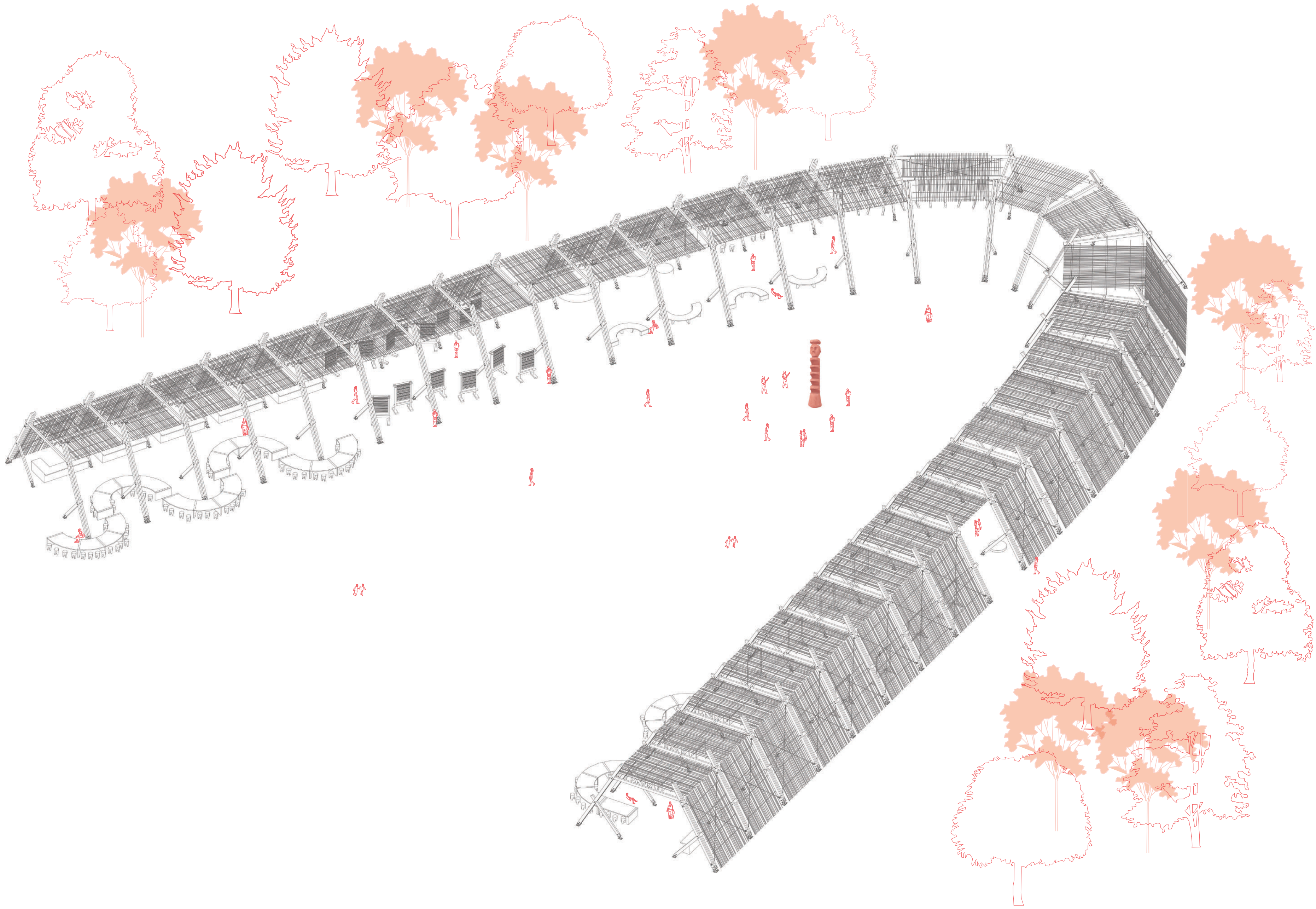
PROYECTO AXONOMETRICA ESC. 1:200
