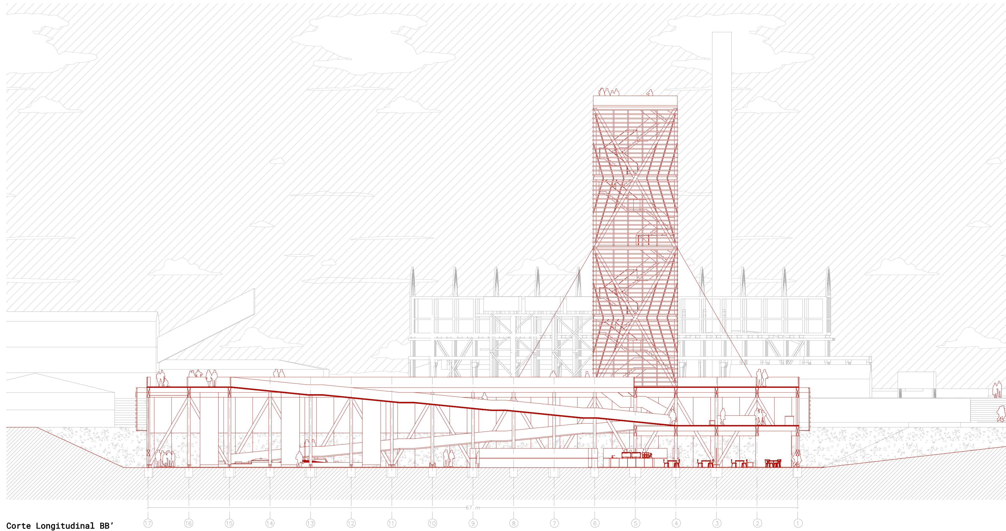
Corte Longitudinal BB' Esc 1:250
