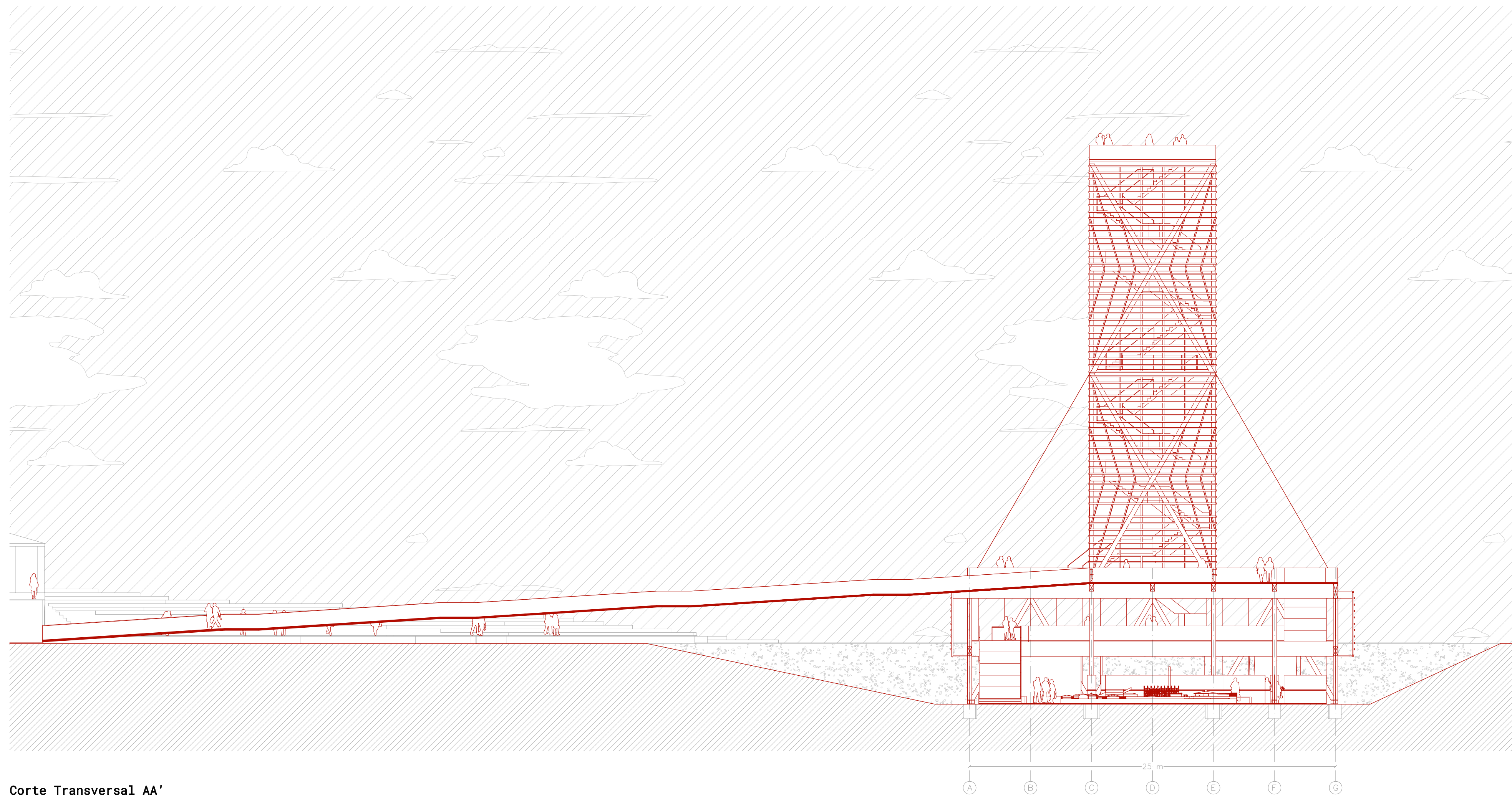
Corte Transversal AA' Esc 1:250
