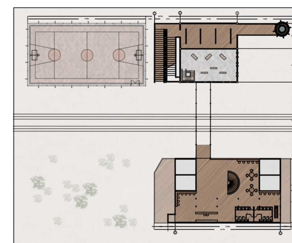
Planta N°3 / Terraza y talleres ESCALA 1/300
