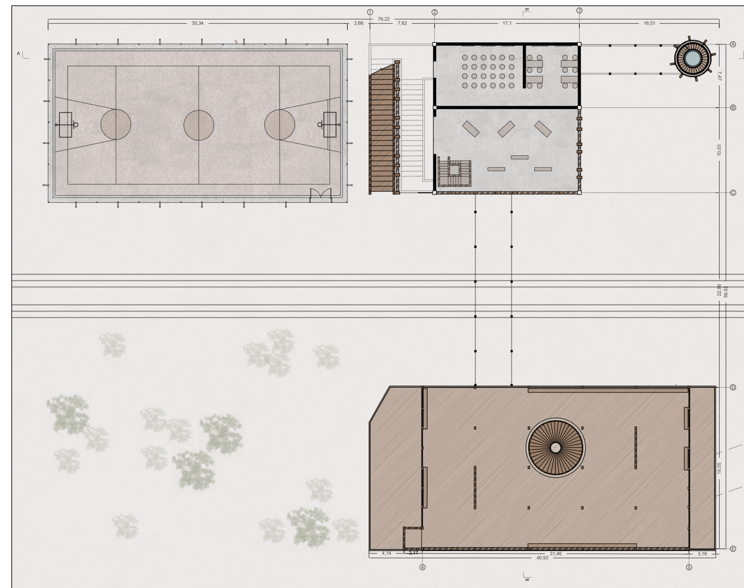
Planta N°2 / Exposiciones ESCALA 1/100
