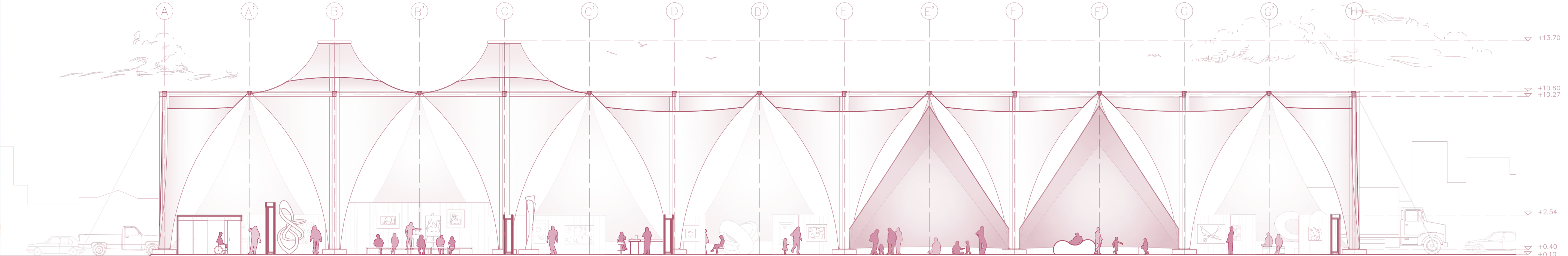
CORTE A - A' ESC 1:175
