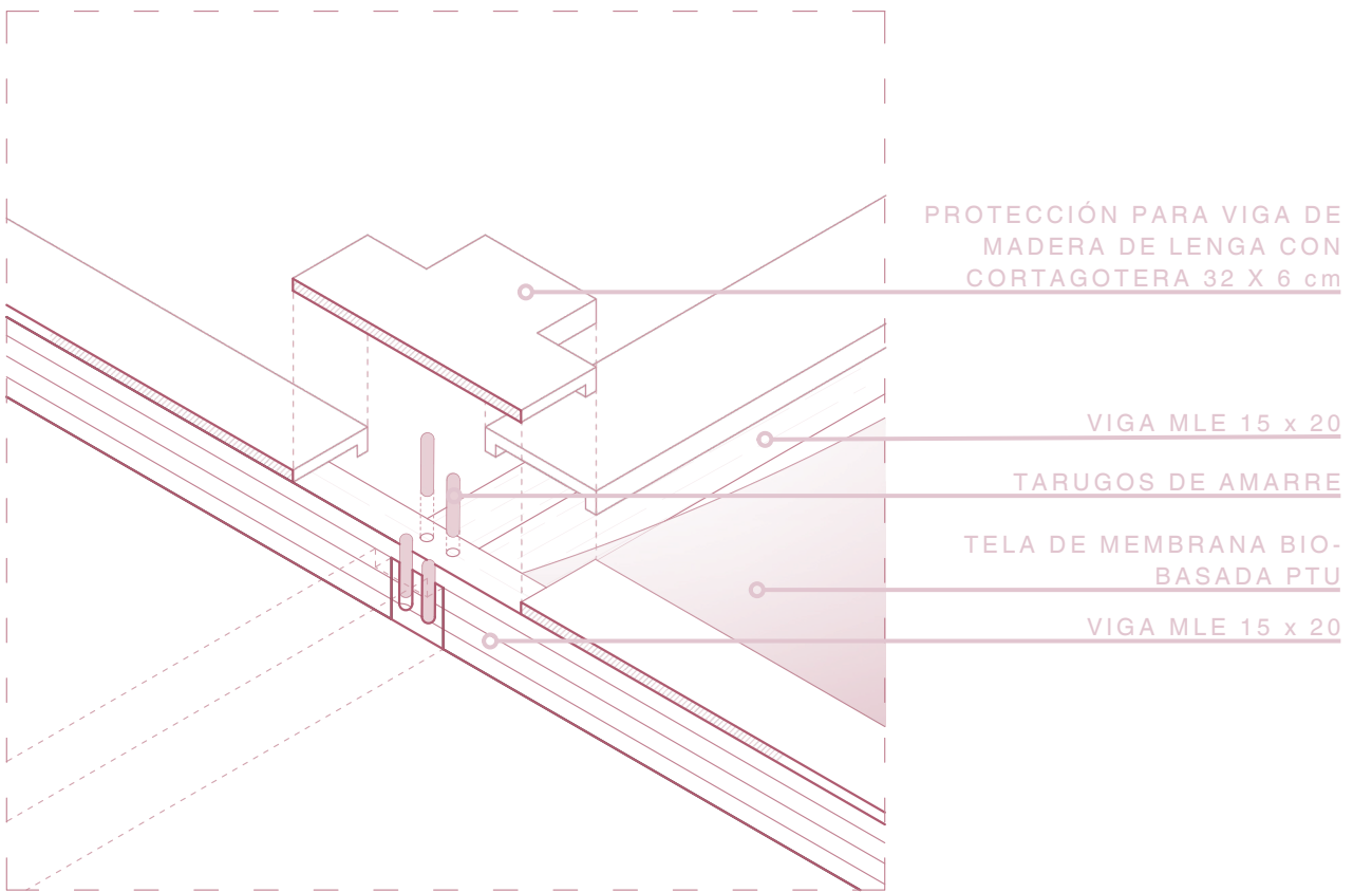
UNIÓN CENTRAL CRUCETA
