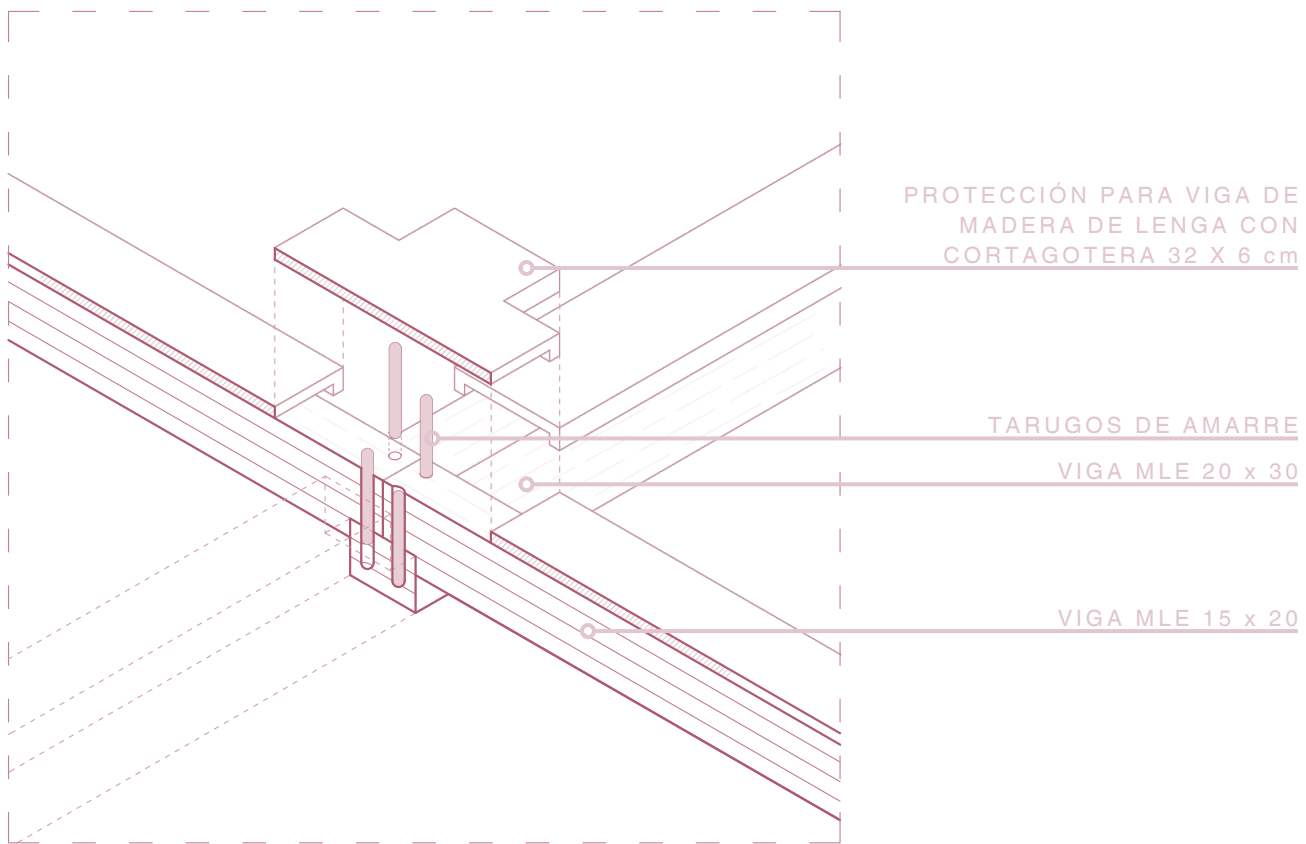
UNIÓN RETÍCULA - CRUCETA
