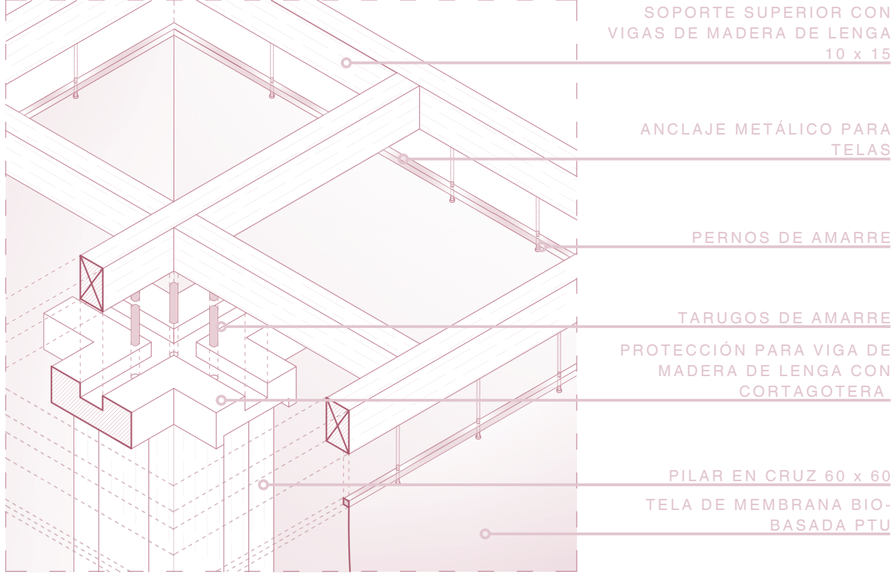
UNIÓN PILAR - SOPORTE SUPERIOR
