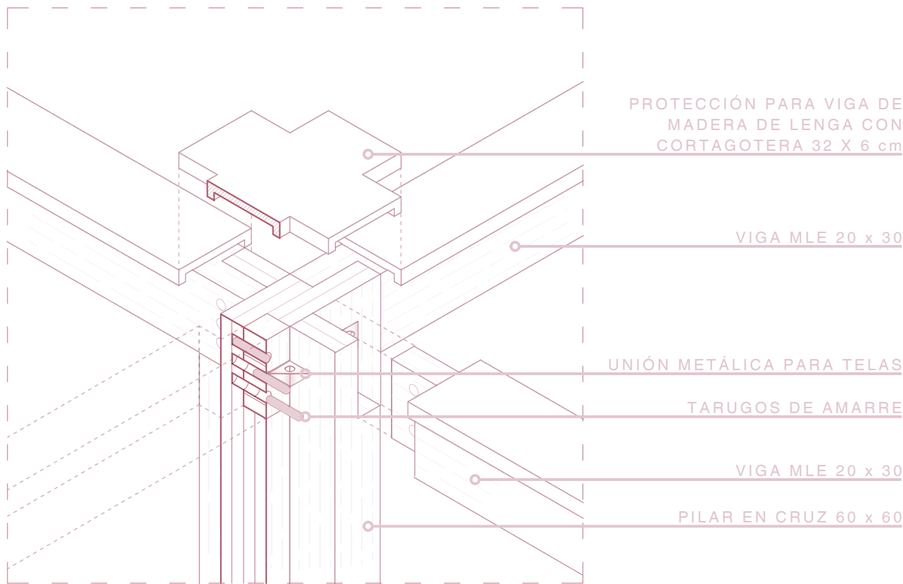
UNIÓN PILAR - VIGA
