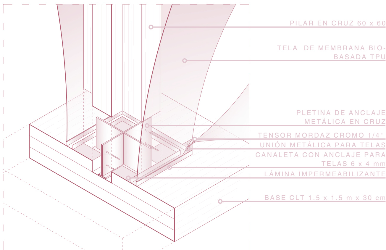
UNIÓN PILAR - BASE
