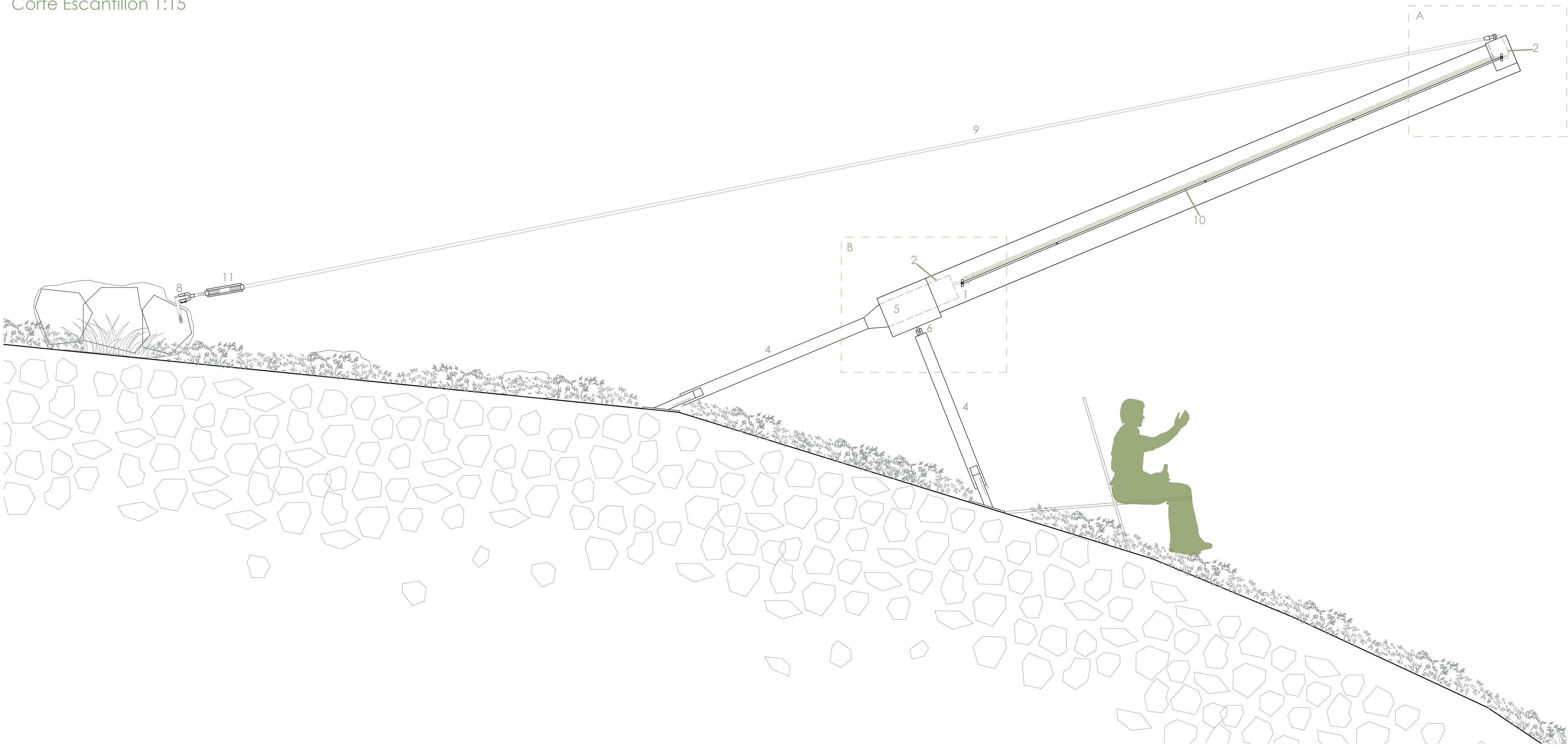
Corte Escantillon 1:15
