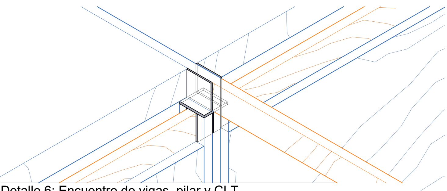
Detalle 6: Encuentro de vigas, pilar y CLT
