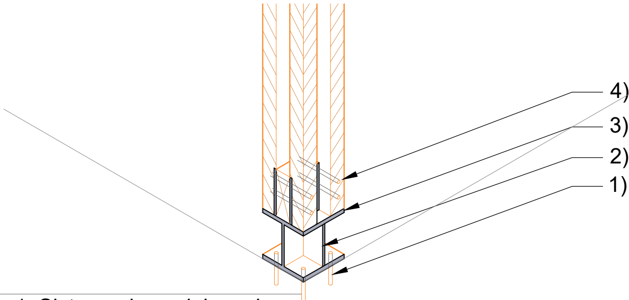
Detalle 1: Sistema de anclaje a piso
