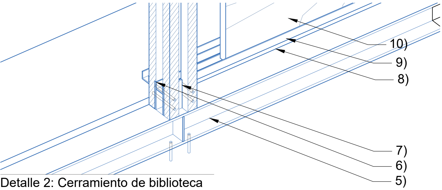
Detalle 2: Cerramiento de biblioteca
