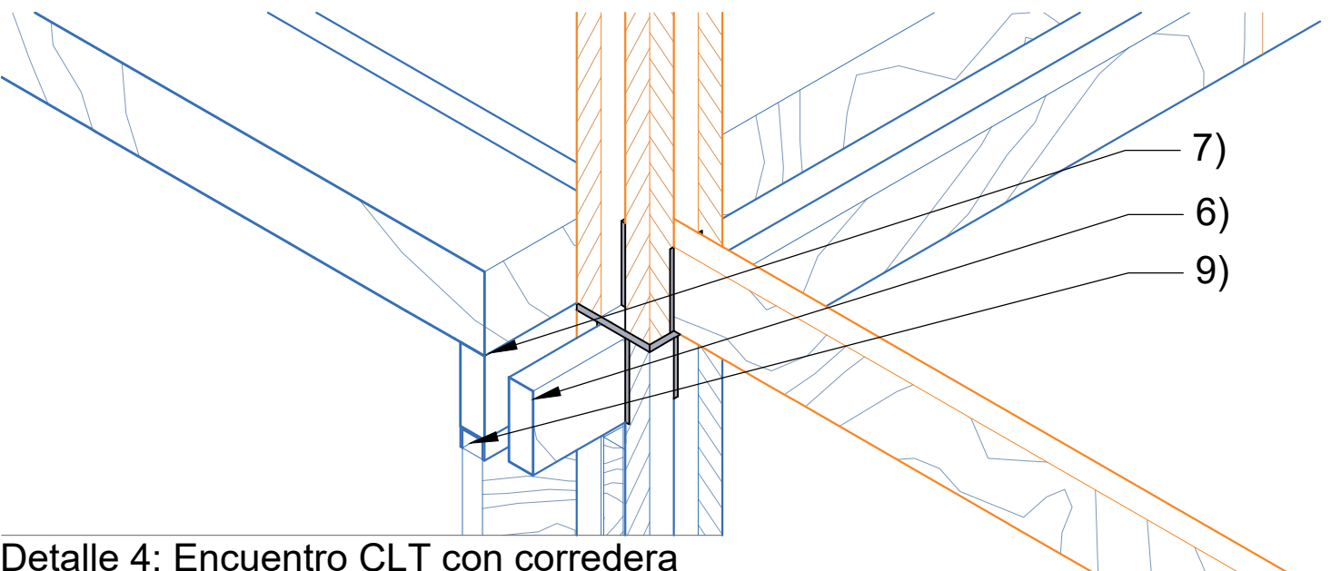
Detalle 4: Encuentro CLT con corredera
