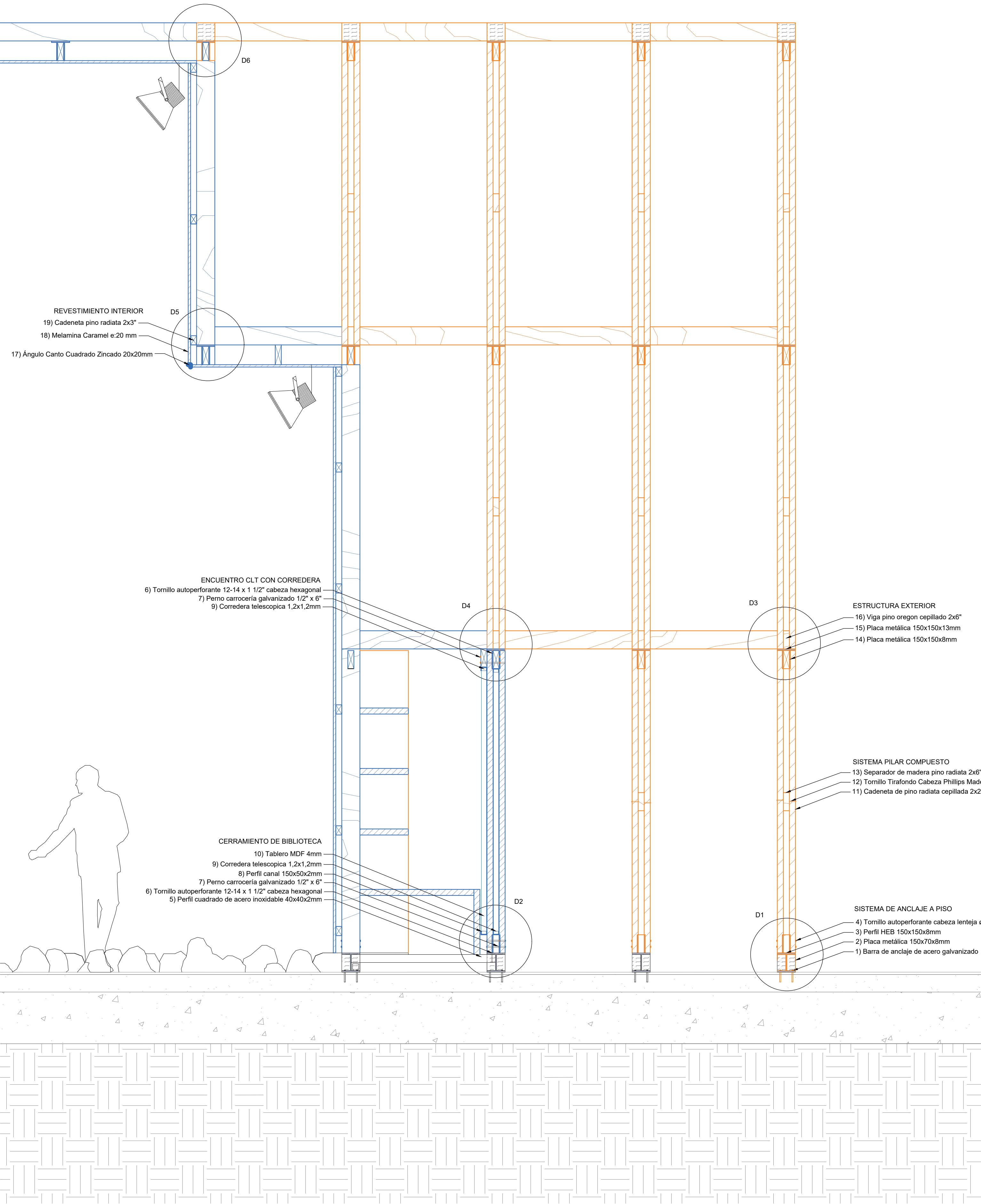
Detalle 6: Encuentro de vigas, pilar y CLT
