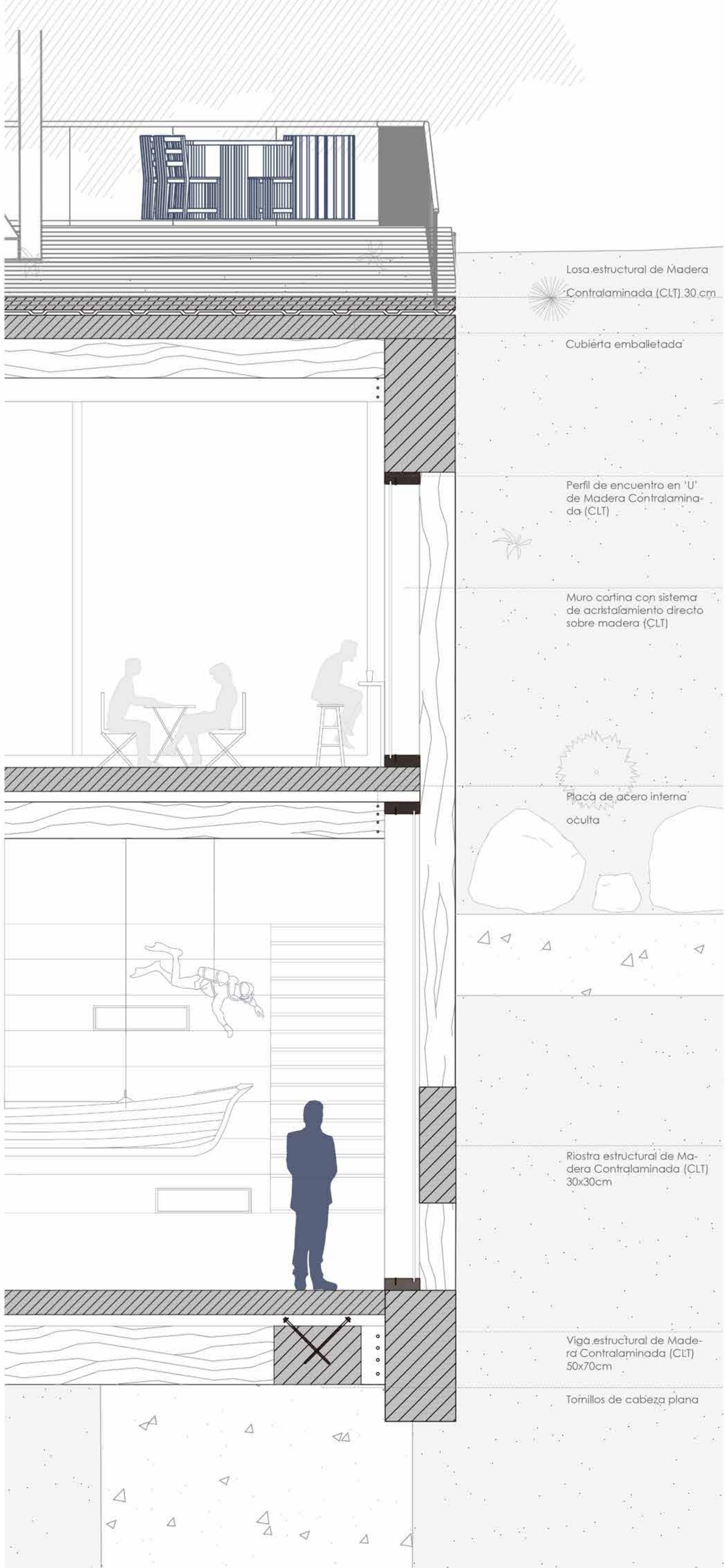
CORTE ESCANTILLÓN
