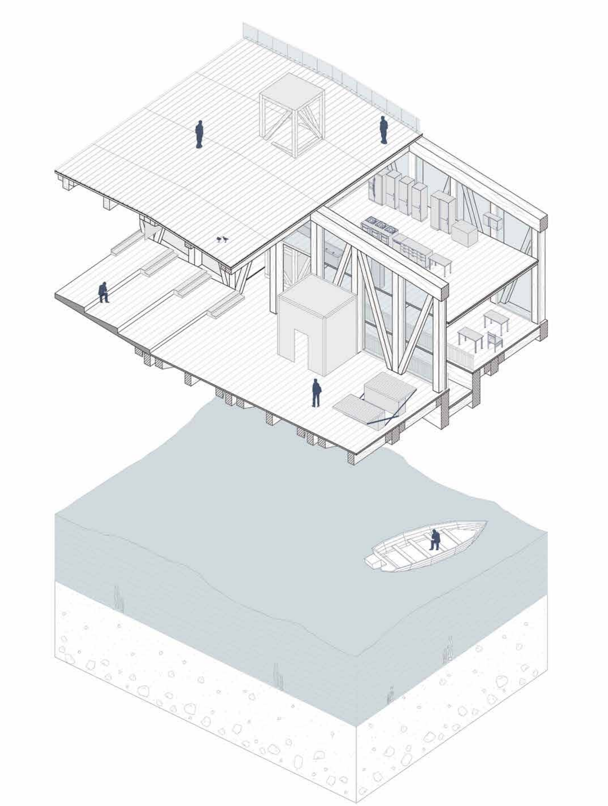
AXONOMÉTRICA ESCANTILLÓN
