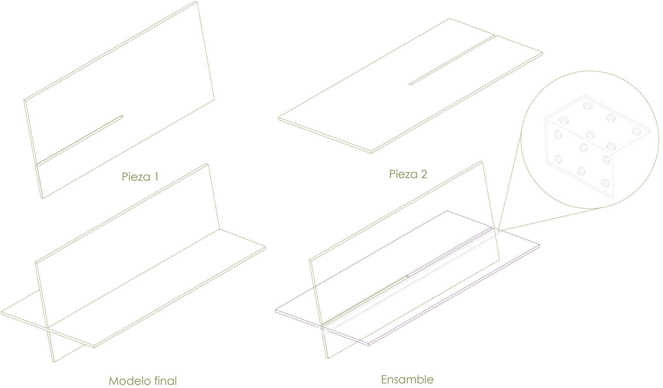
Sistema constructivo mobiliario
