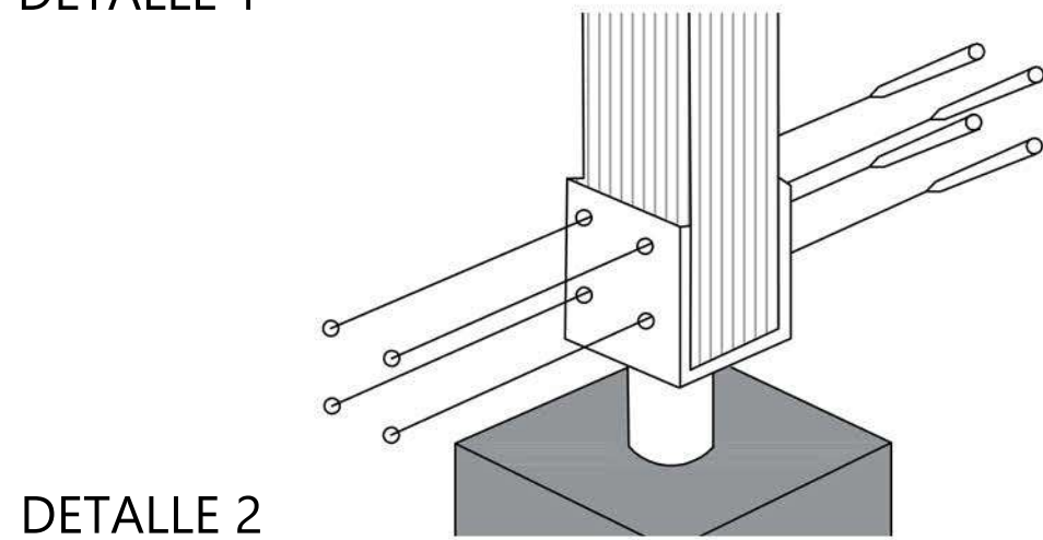
DETALLE 2
