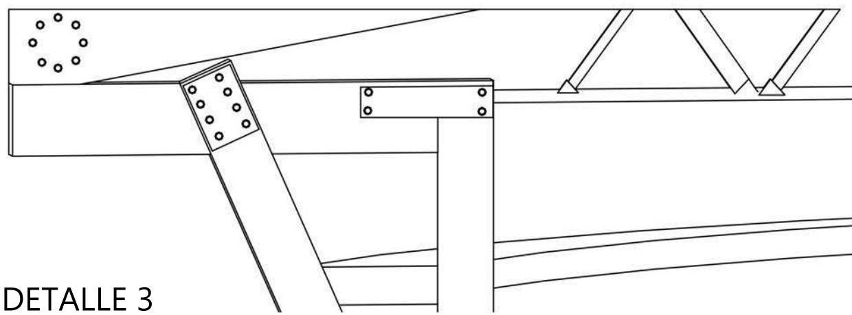
DETALLE 3
