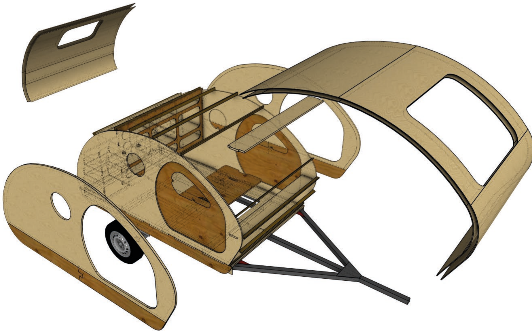
Modelo 3D con partes que conforman la cabina y sus zonas de uso.
