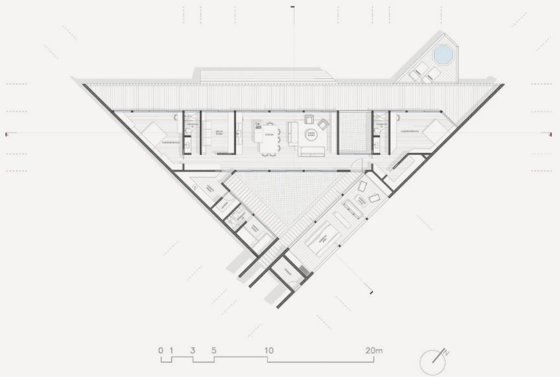
PLANTA ARQUITECTURA
