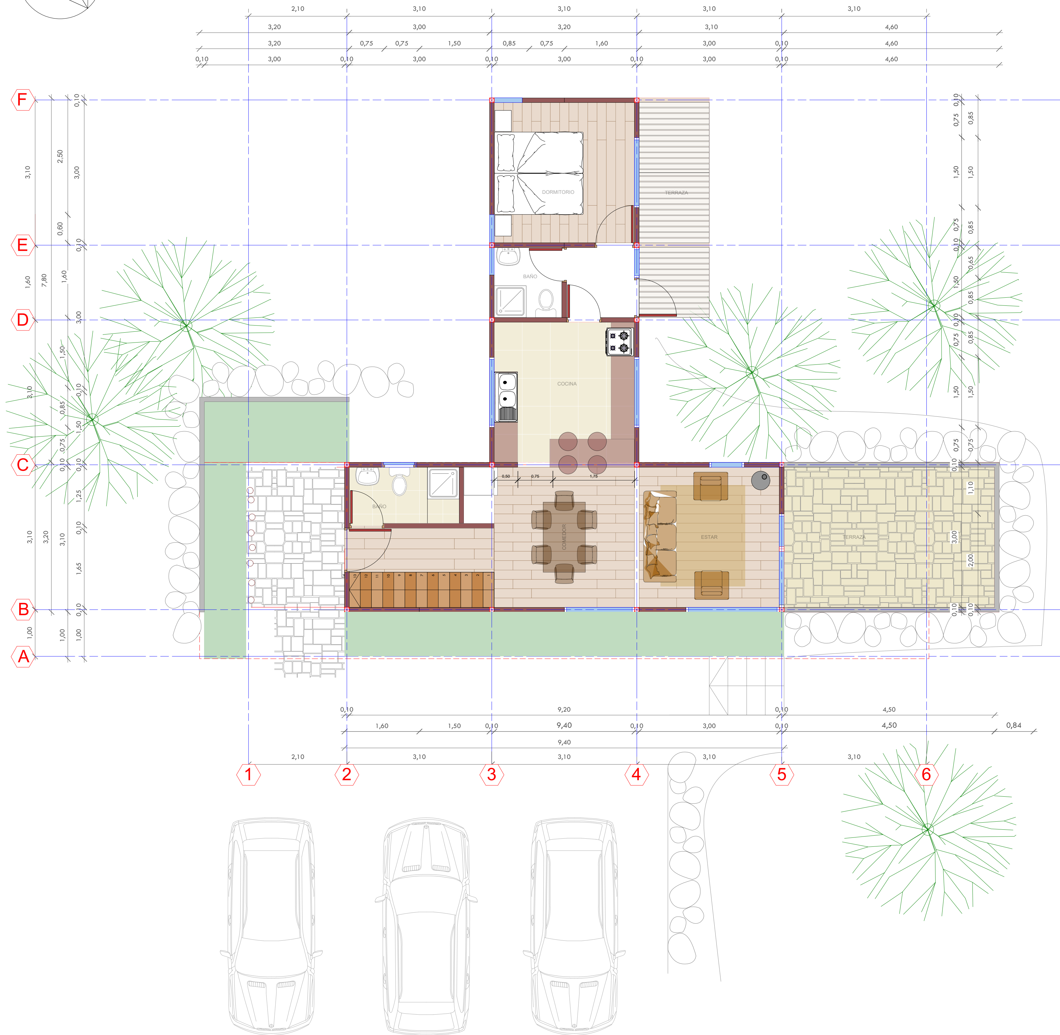
PLANTA ARQUITECTURA PRIMER NIVEL ESC. 1/50
