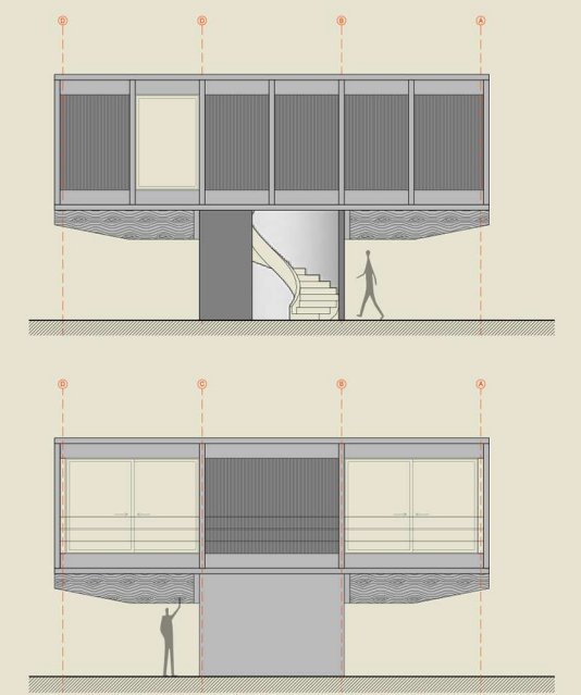
ELEVACIONES ORIENTE Y PONIENTE
