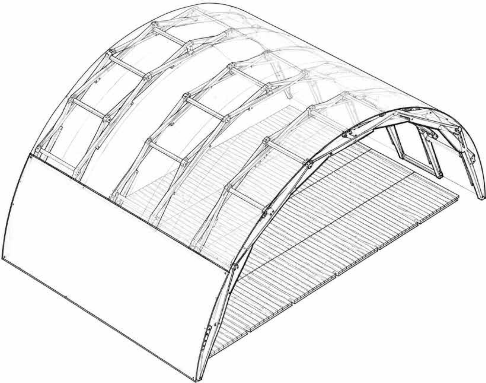
MEDIDAS DE REFERENCIA DE UN GALPÓN MODULAR
