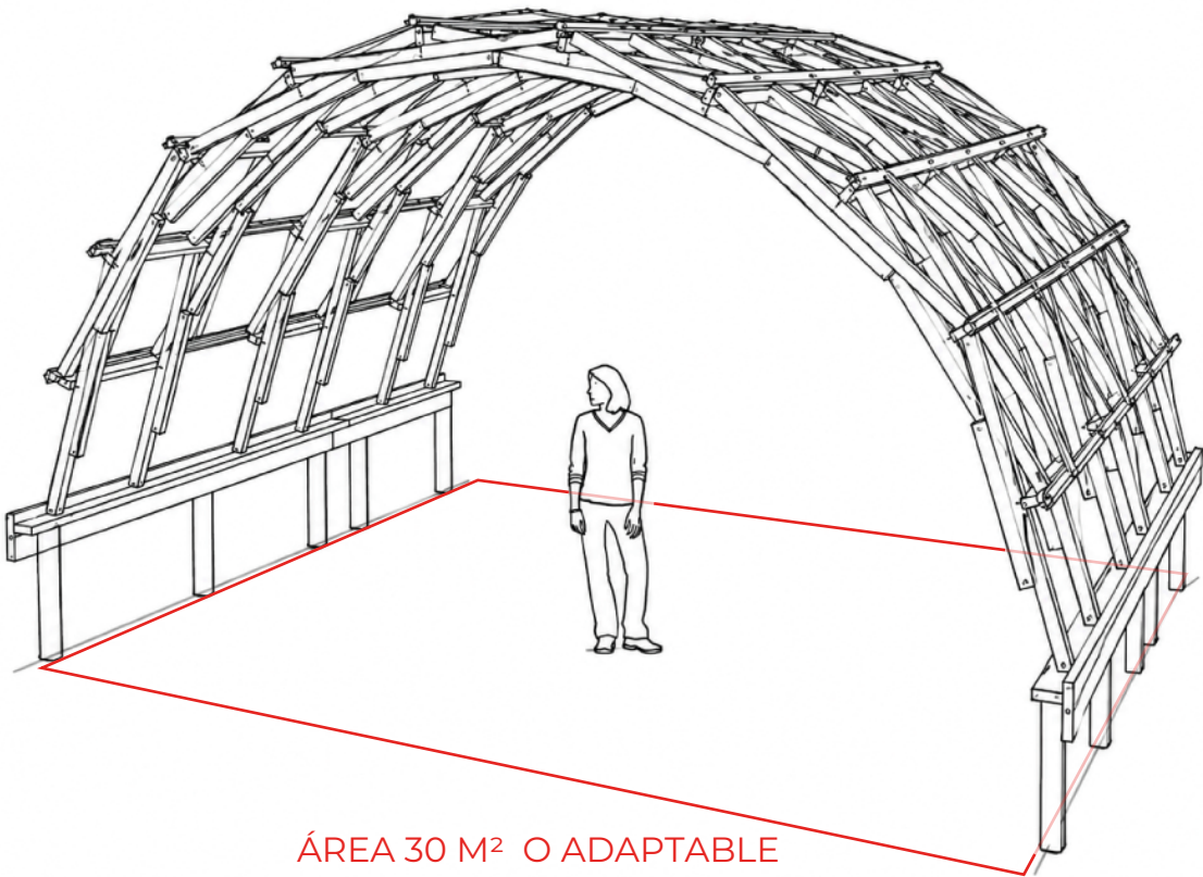
MEDIDAS DE REFERENCIA DE UN GALPÓN MODULAR
