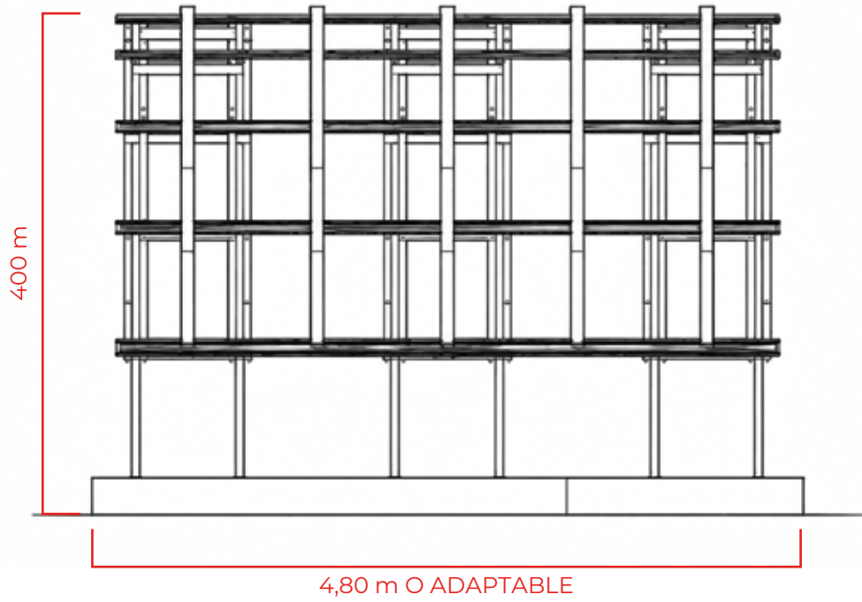
ELEVACIÓN LATERAL
