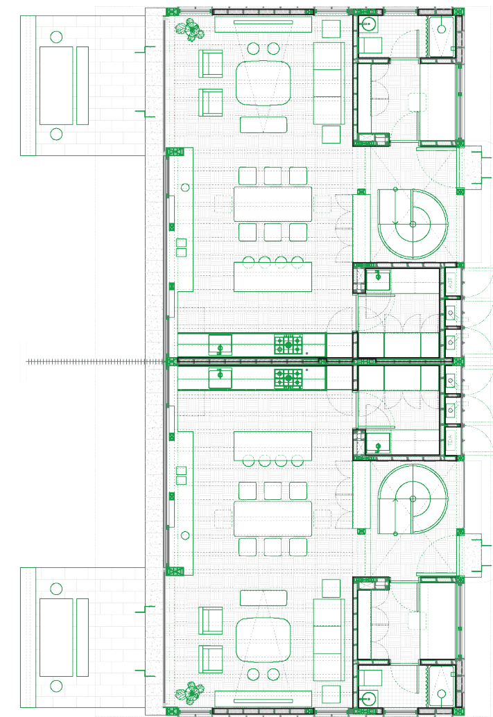
Planta Nivel 1
