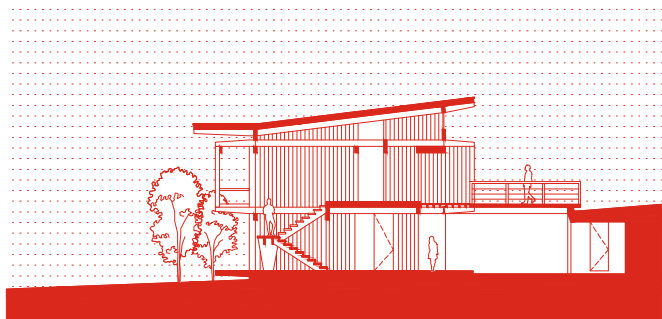
Corte C-C
