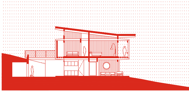
Corte B-B
