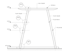
ELEVACIÓN MARCO TIPO
