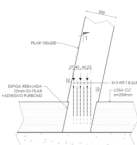
DETALLE 1
