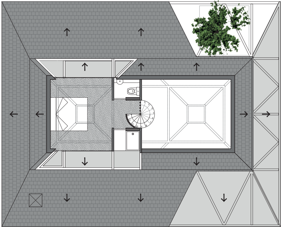
PLANTA PISO 2
