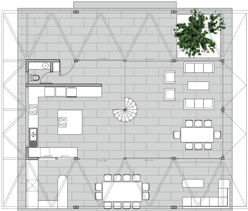
PLANTA PISO 1
